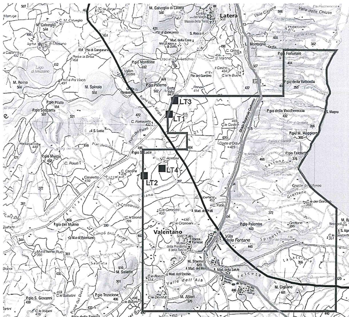
Figura 1: Limite del permesso “Latera Pilota (linea rossa), limite del bacino idrogeologico del Lago di Bolsena (linea blu) e limite del bacino idrogeologico del Lago di Bolsena (linea verde). Sono indicate le posizioni dei pozzi di produzione LT1 e LT3, e dei pozzi di reiniezione (LT2 e LT4).
