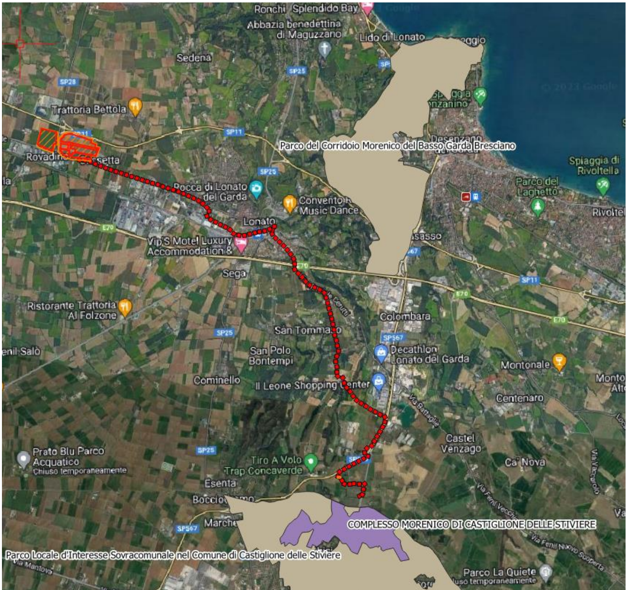
Figura 5: inquadramento su base google maps dell'impianto agri voltaico (nord-ovest) di tutto il percorso di cavidotto interrato sotto strada (linea tratteggiata rossa) e della sotto stazione elettrica (in zona sud). Quest'ultima opera, accessoria e funzionale all'intero impianto, dista poco più di 400 m dal SIC "Complesso morenico di Castiglione delle Stiviere".
