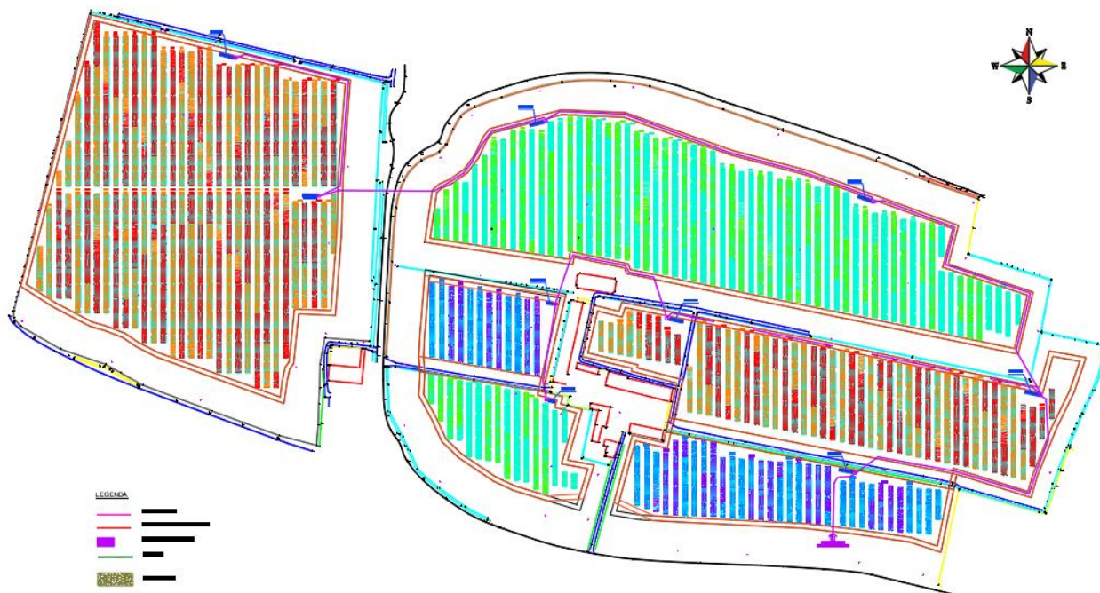
Figura 3: Planimetria di massima della disposizione dei diversi pannelli fotovoltaici sul territorio aziendale. Lungo il perimetro le fasce di rispetto dedicate alla mitigazione paesaggistica e ambientale dell'intervento (siepi-filari).
