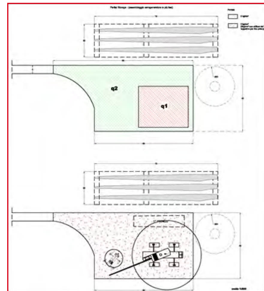
Fig. 2 - schema tipo di piazzola tipologica in fase di cantiere per il montaggio dell'aerogeneratore (da stralcio progettuale)
