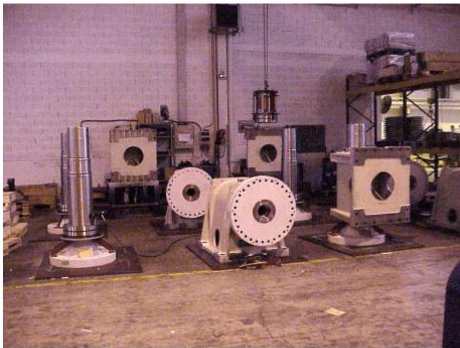
Figura 9: asse di bassa velocità
