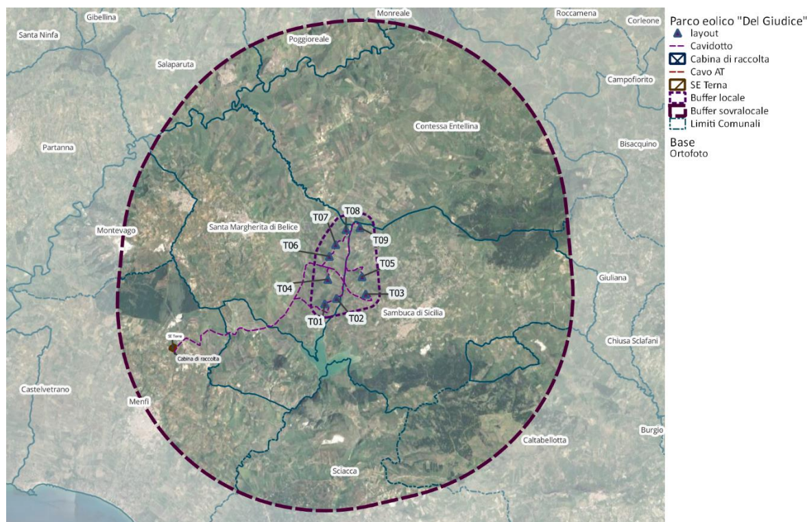
Figura 2. Layout di impianto su base ortofoto
