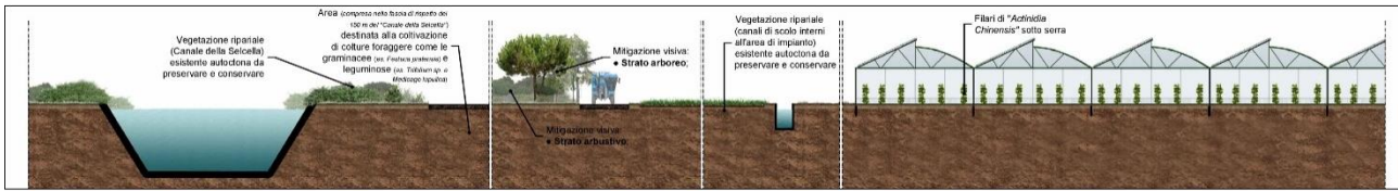
Figura 20 – Sezione longitudinale tipo degli interventi progettuali proposti
