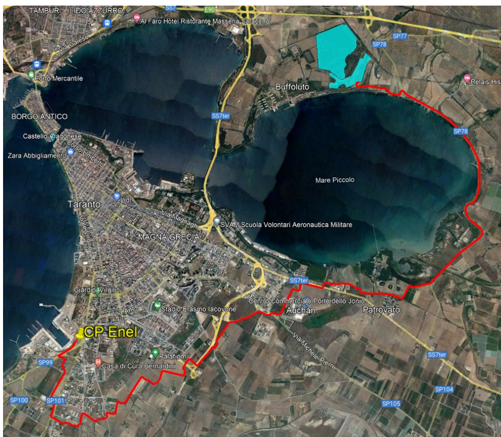
Fig. 1. Planimetria su ortofoto del progettato impianto Fotovoltaico: in colore ciano viene indicata l'area del generatore fotovoltaico, in rosso il cavidotto dorsale MT di collegamento tra il generatore e la Sottostazione Produttore, ubicata in prossimità della Cabina Primaria Enel
