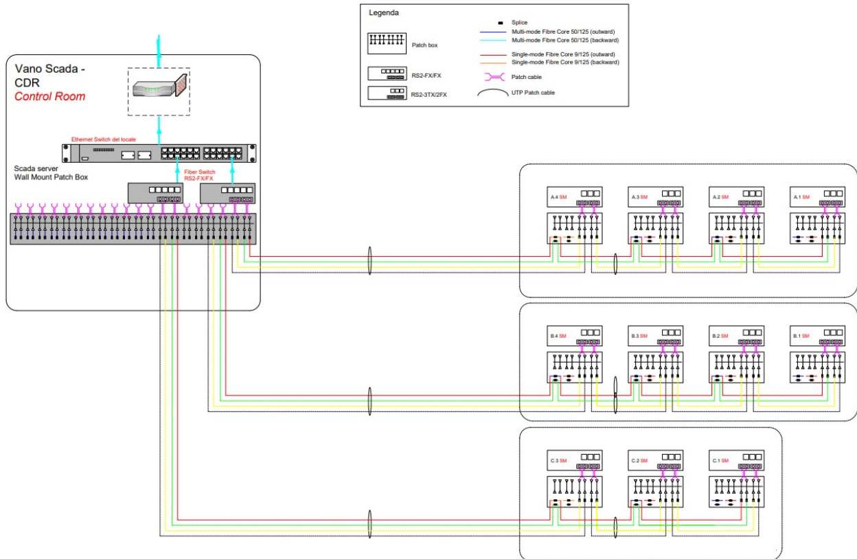
Fig. 11. Schema a blocchi per l'interconnessione degli impianti.
