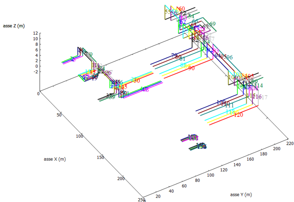
Figura 5 – Schematizzazione degli elementi attivi all'interno del programma di calcolo
