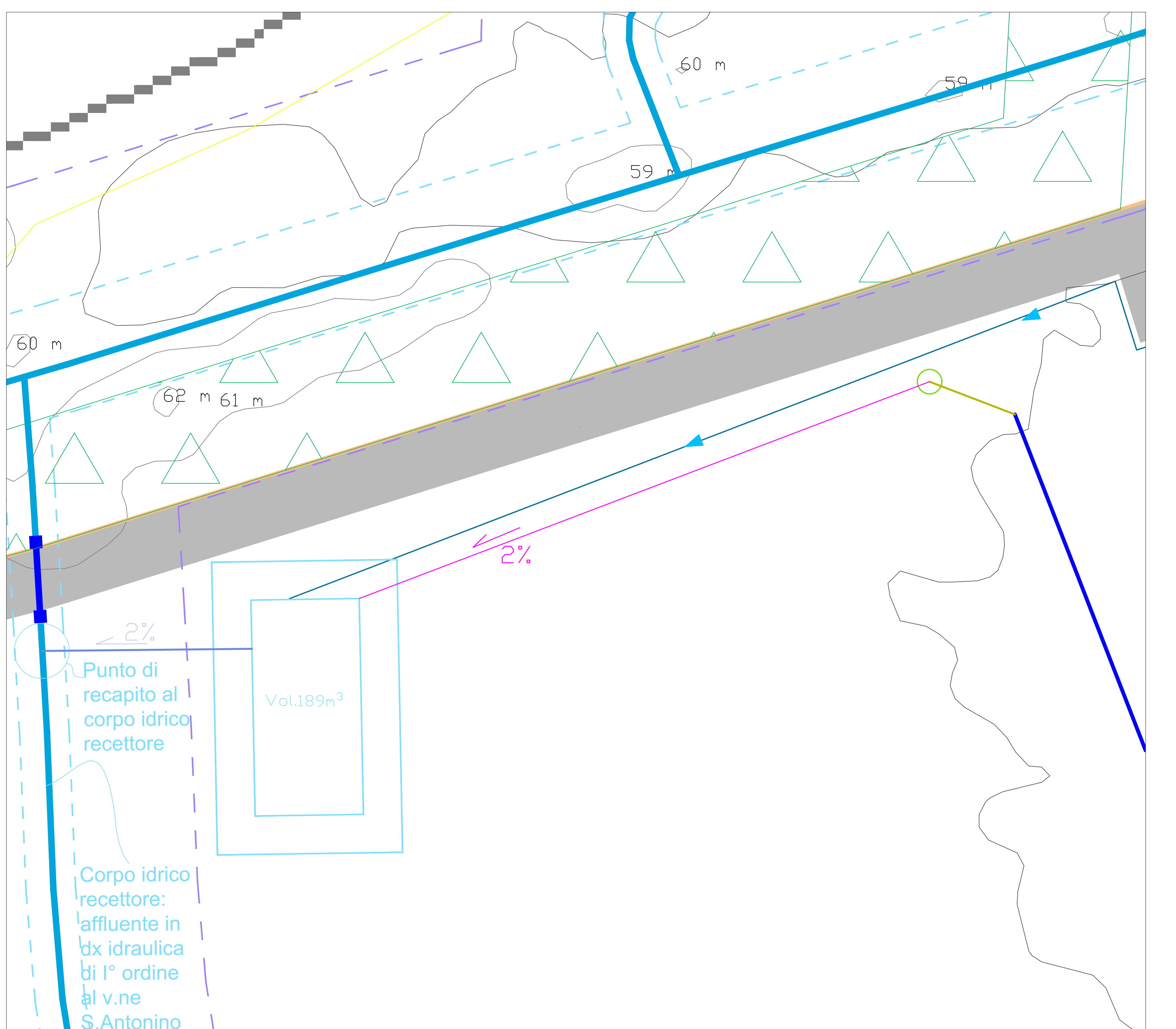
Lotto C.2 - Scala 1:500
