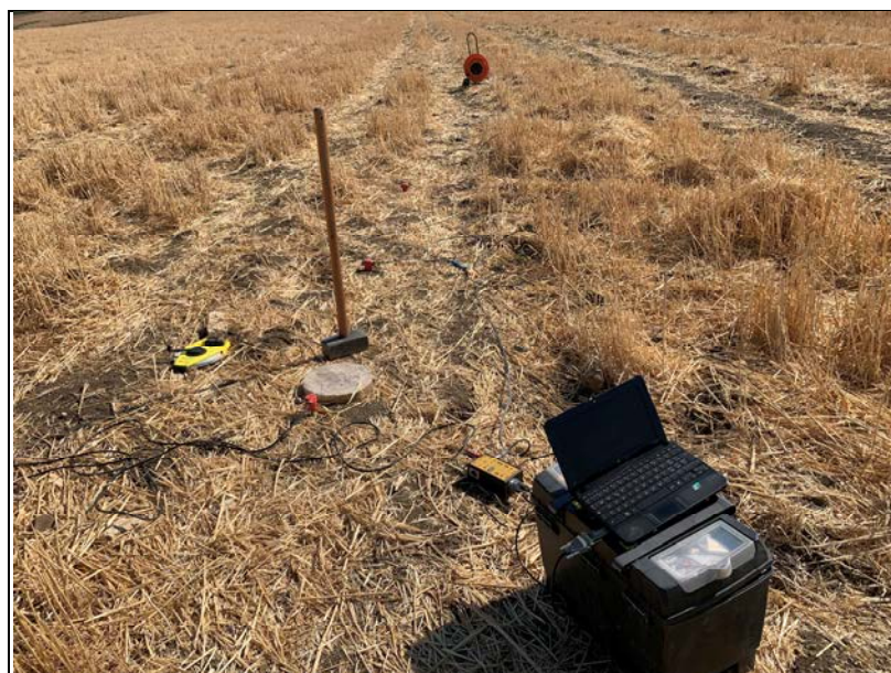
Stesa sismica ST 1
