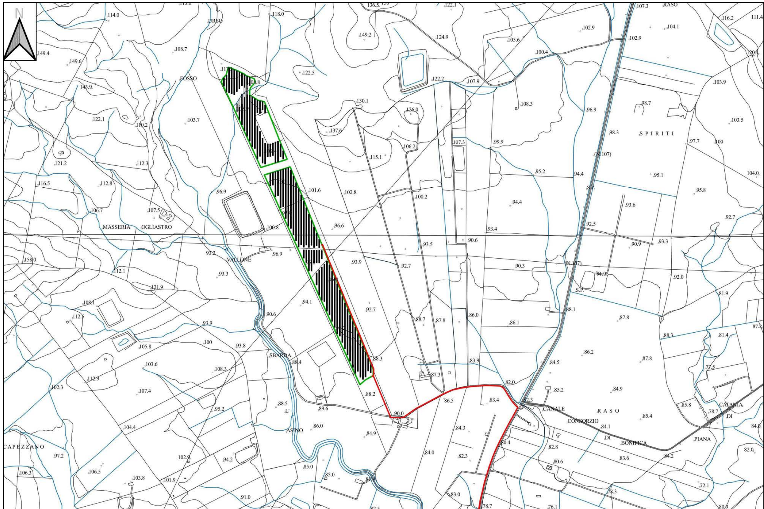
Stralcio aerofotogrammetrico in scala 1:10.000 dell'area Nord dell'impianto
