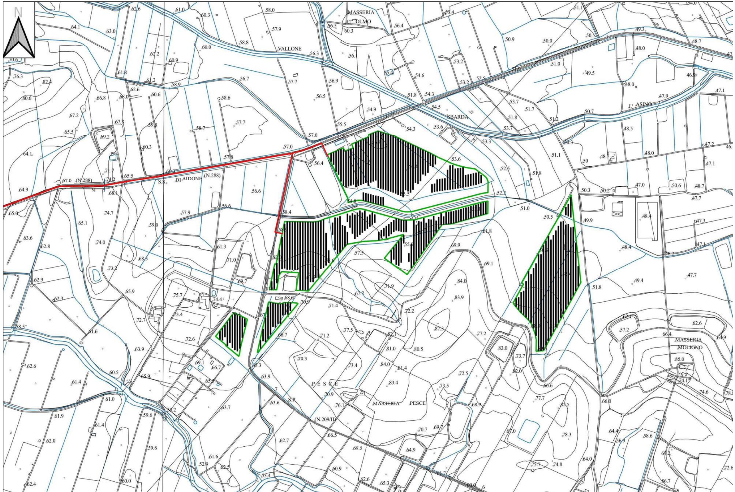
Stralcio aerofotogrammetrico in scala 1:10.000 dell'area Sud dell'impianto
