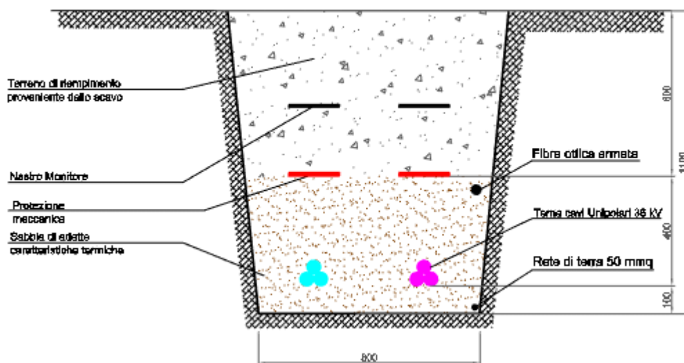
Figura 3 Sezione tipo cavidotto interrato AAT
