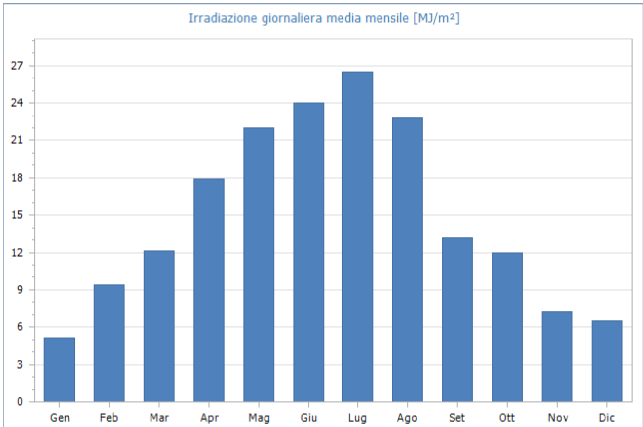
Fig. 1: Irradiazione giornaliera media mensile sul piano orizzontale [MJ/m 2 ]- Fonte dati: UNI 10349:2016 - Stazione di rilevazione: Montefiascone
