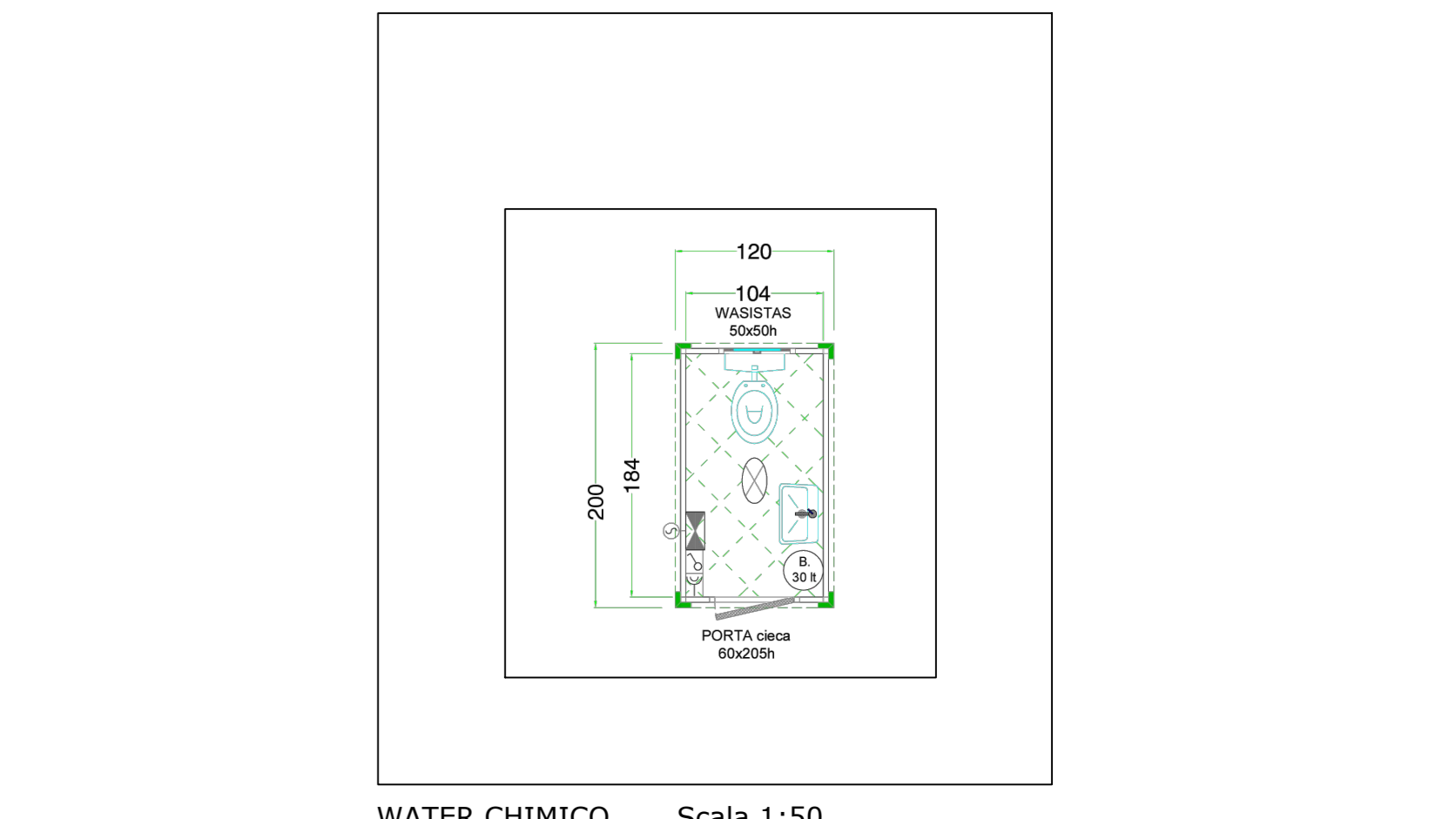
WATER CHIMICO Scala 1:50
