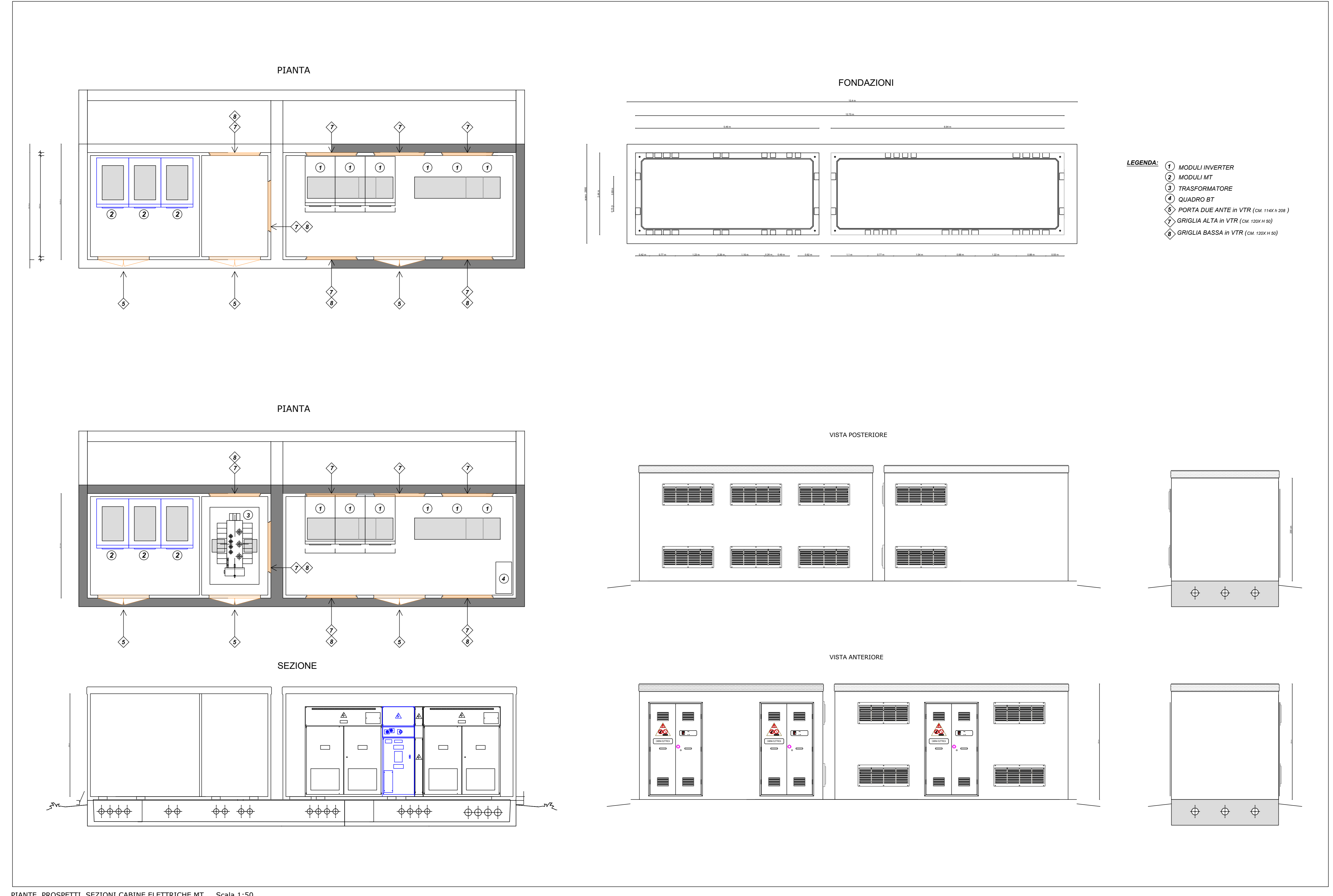
PIANTE, PROSPETTI, SEZIONI CABINE ELETTRICHE MT Scala 1:50
