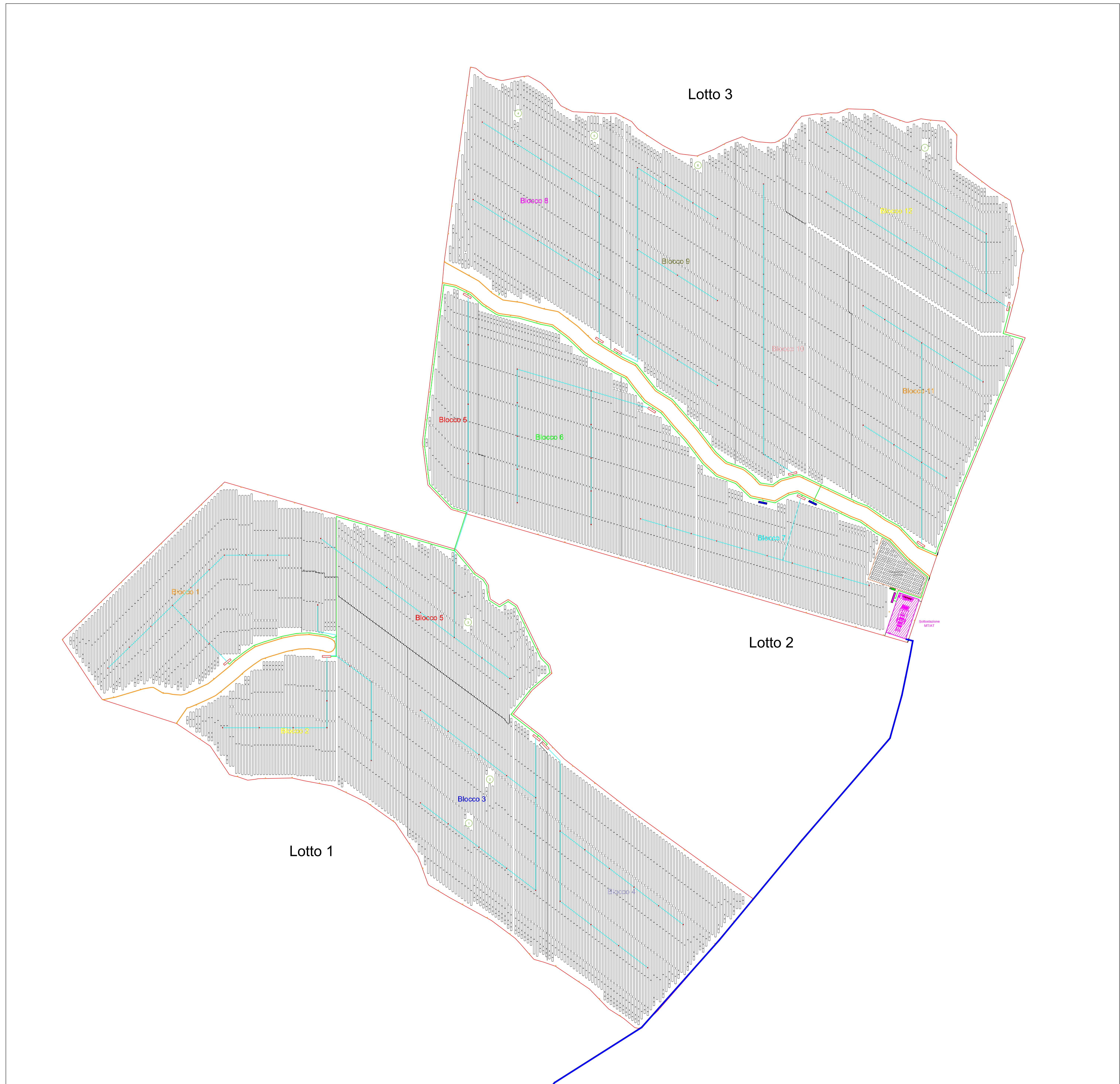
Planimetria canalizzazioni Sc 1:2000
