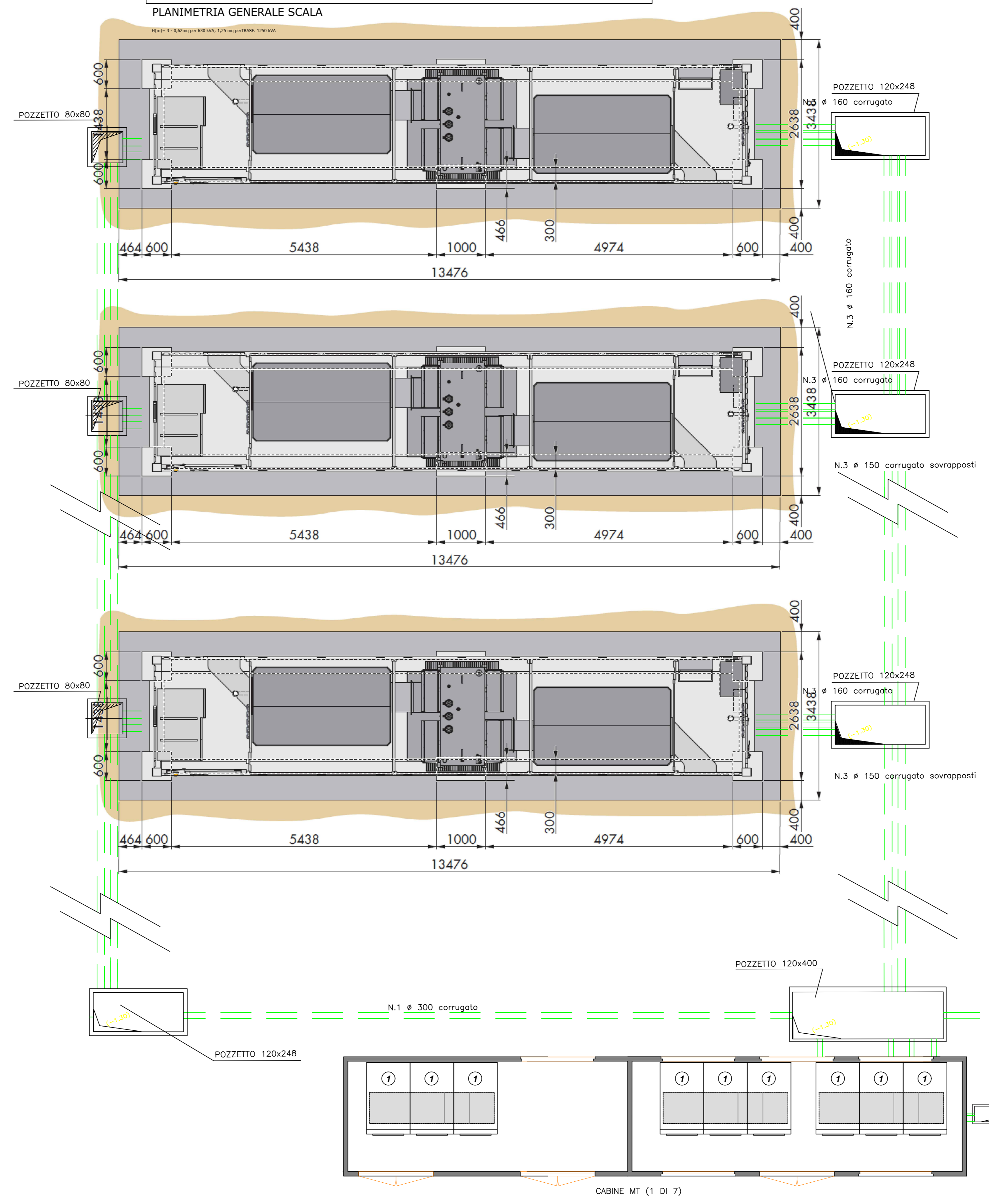
CABINA INVERTER Scala 1:50
