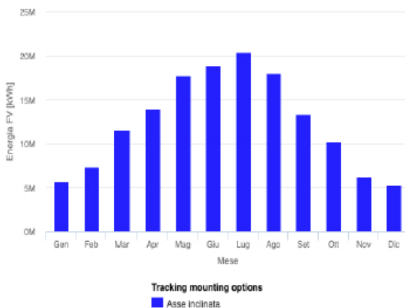
Energia mensile da sistema FV ad inseguimento:
