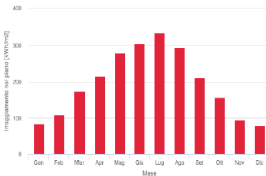
Irraggiamento mensile nel piano di inseguimento:
