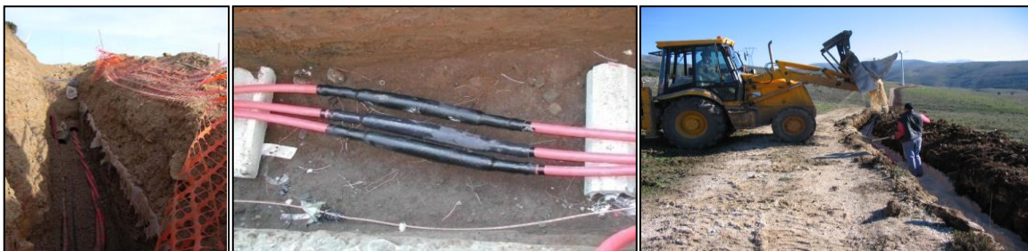
Figura 20: Posa cavi interrati
