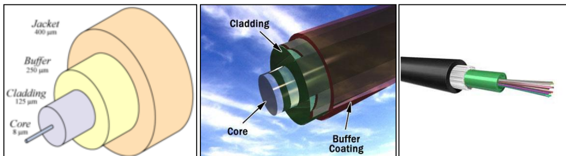
Figura 10: Fibre ottiche
