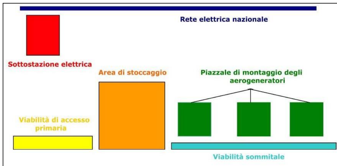
Figura 15: Organizzazione aree del cantiere
