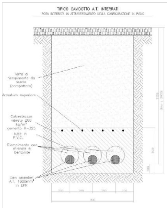
Figura 5: Posa tipo cavo AT
