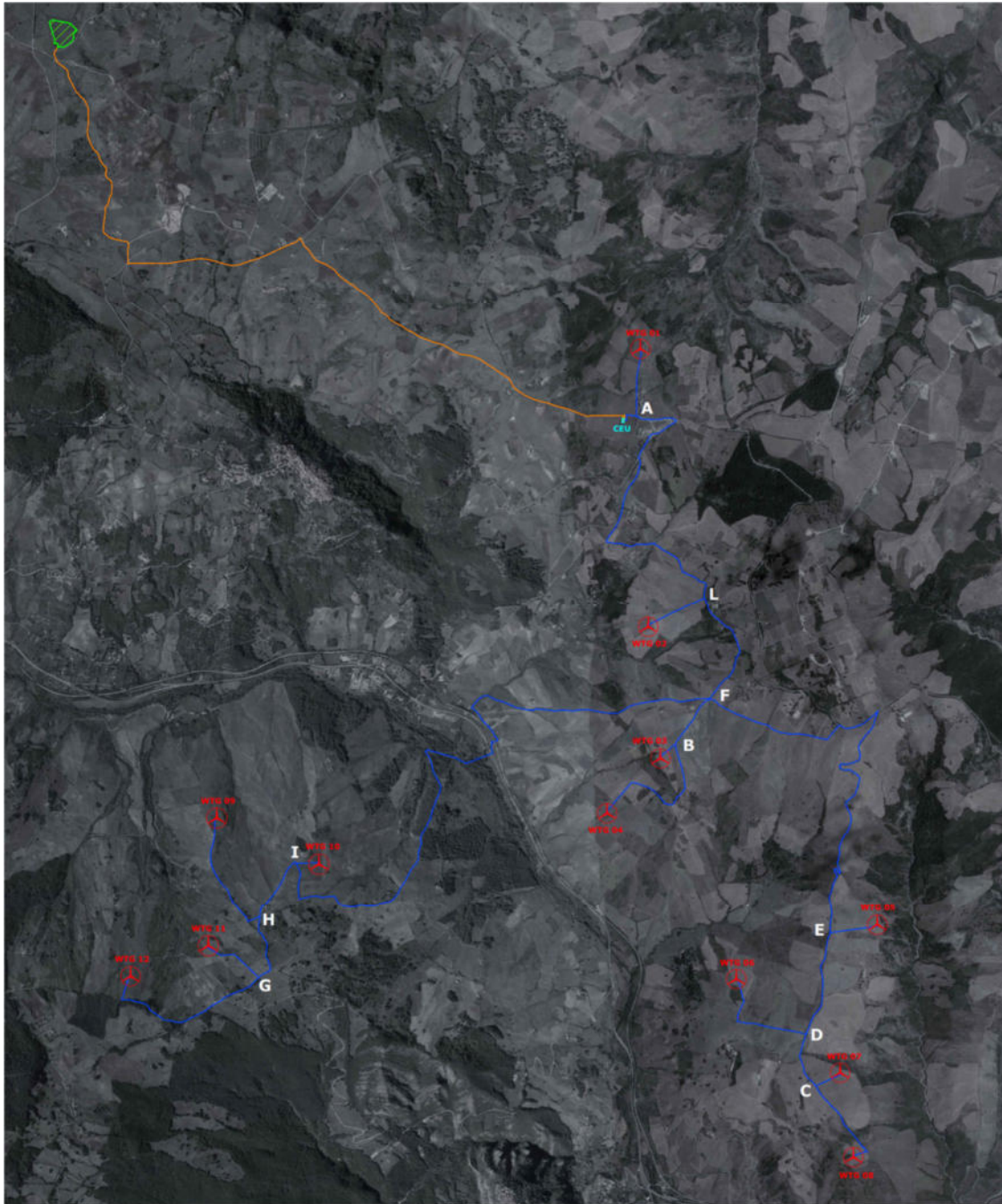
Figura 3 Rappresentazione del Layout delle tratte della distribuzione elettrica a 36 kV
