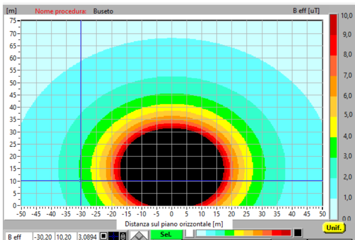
Figura 4. Profilo laterale del campo magnetico a quota conduttori I=870A
