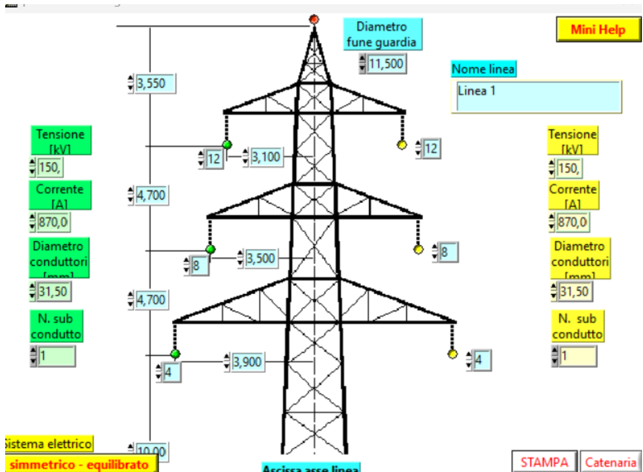
Fig.1 Configurazione di calcolo tratti linea DT
