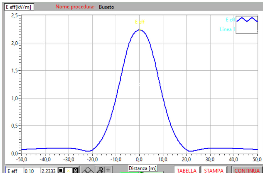
Figura 3. Profilo laterale del campo elettrico ad 1,5 m dal suolo E=2,23 kV/m;
