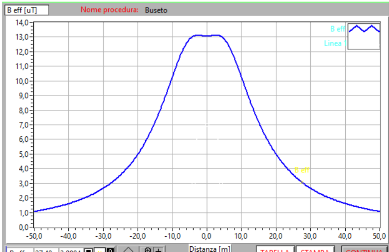
Figure 2. Profilo laterale dell'induzione magnetica ad 1,5 m dal suolo B=13 \mu T
