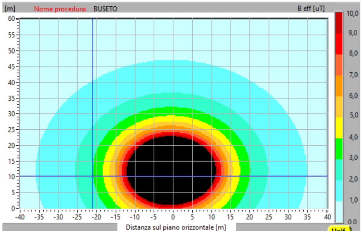
Figura 4. Profilo laterale del campo magnetico a quota conduttori I=870A
