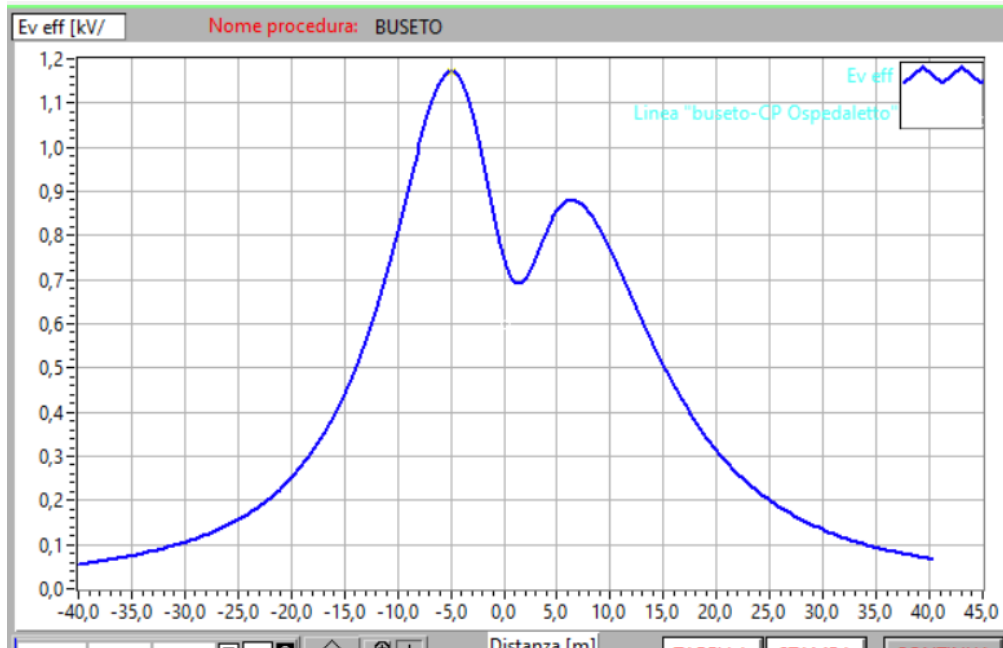
Figura 3. Profilo laterale del campo elettrico ad 1,5 m dal suolo E=1,17 kV/m
