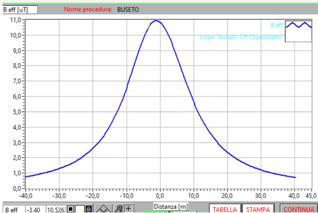
Figure 2. Profilo laterale dell'induzione magnetica ad 1,5 m dal suolo B=11 \mu T
