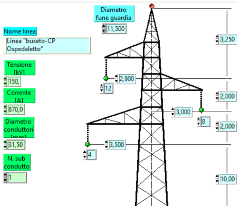
Fig.1 Configurazione di calcolo tratti linea ST
