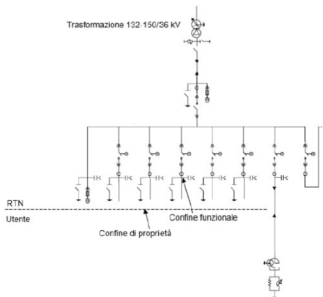
Figura 1 - Schema di connessione esemplificativo a 36 kV
