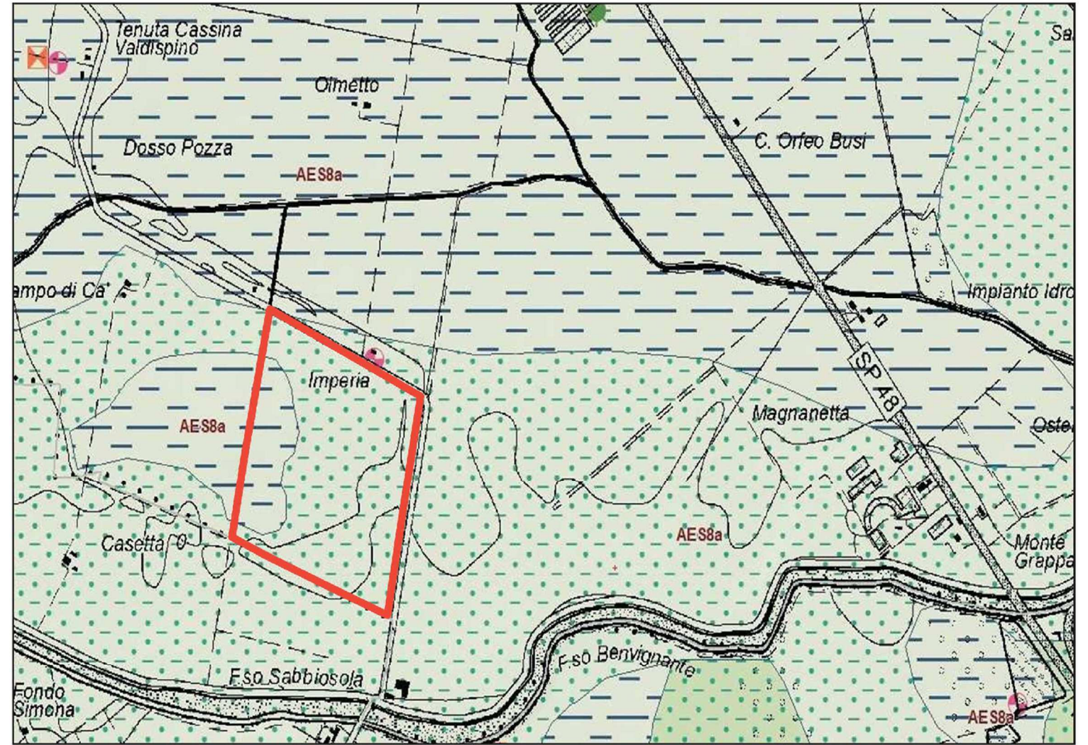
Stralcio Carta Geologica 1:10.000
