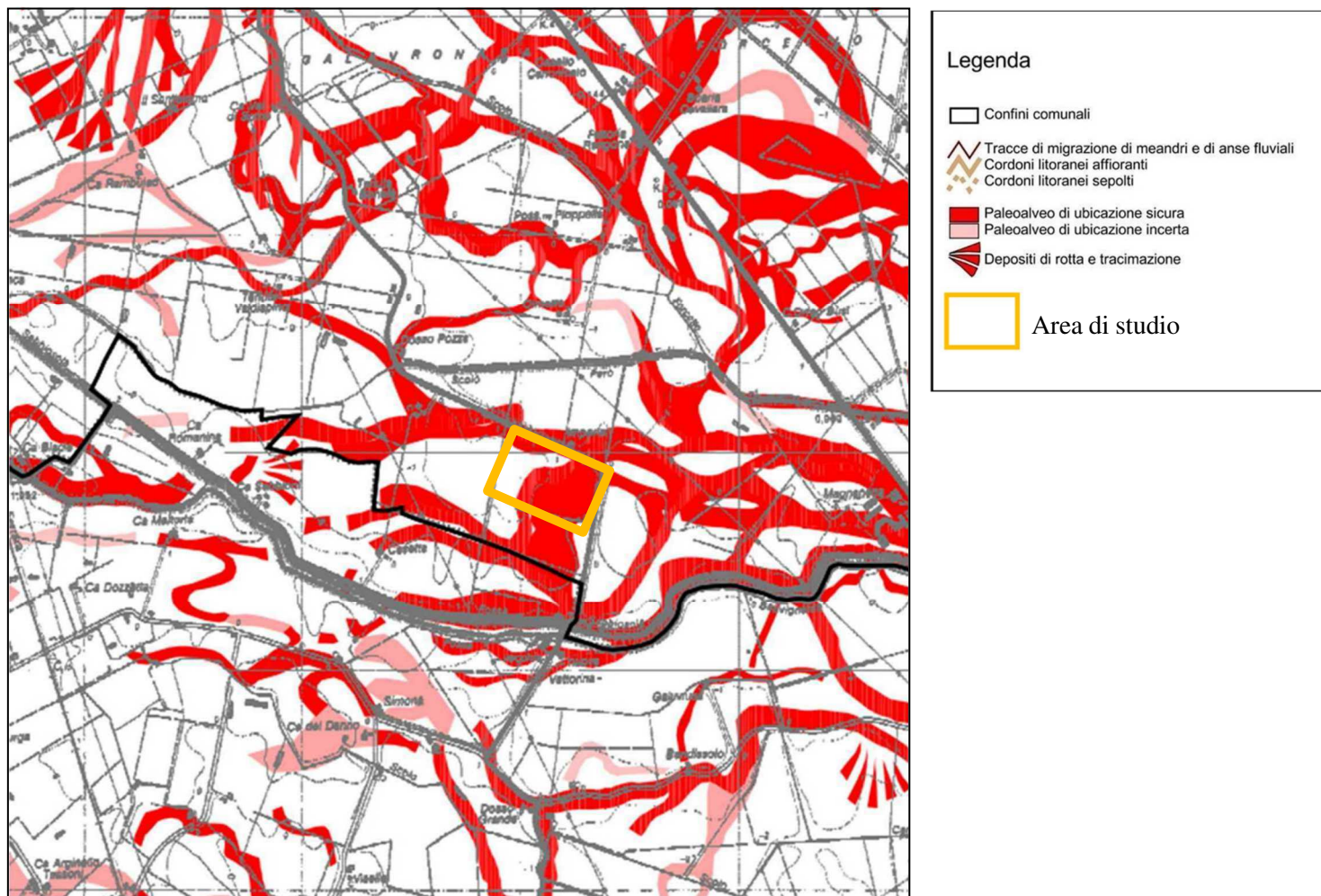
Figura 5: Stralci Carta geo morfologica del Comune di Portomaggiore –scala 1:5.000.
