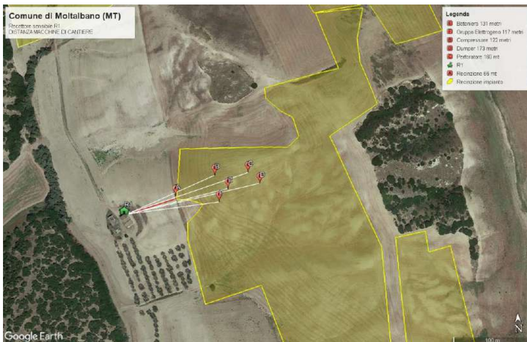
Figura 3 - distanziamento medio macchinari dal recettore sensibile R1
