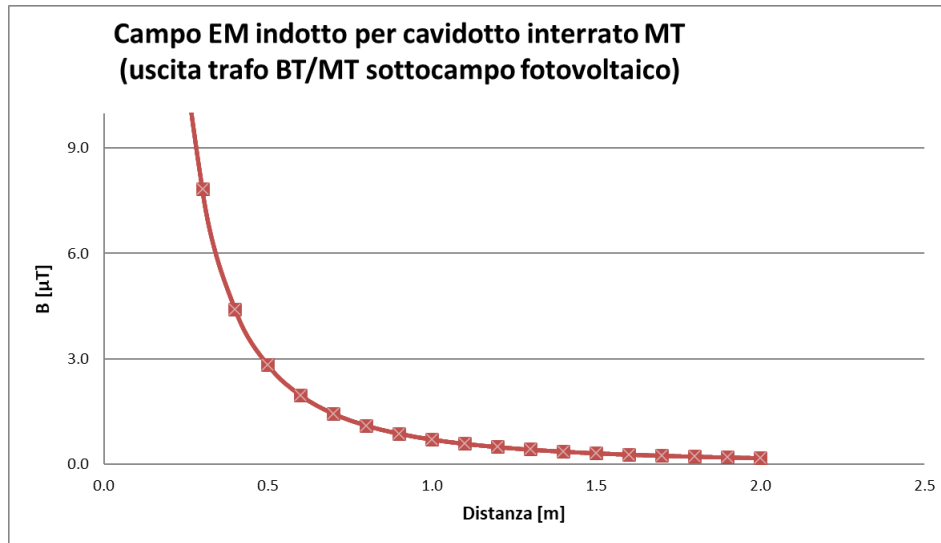
Figura 3 – Andamento dell’induzione E.M. per conduttori in MT in uscita dalle power stations in funzione della distanza dal conduttore (Norma CEI 106-12)
