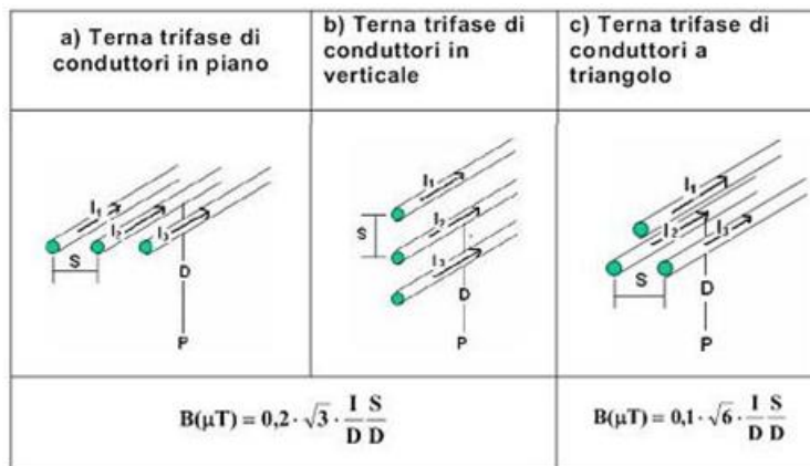
Figura 4 - Calcolo semplificato campo magnetico indotto (Norma CEI 106-12)
