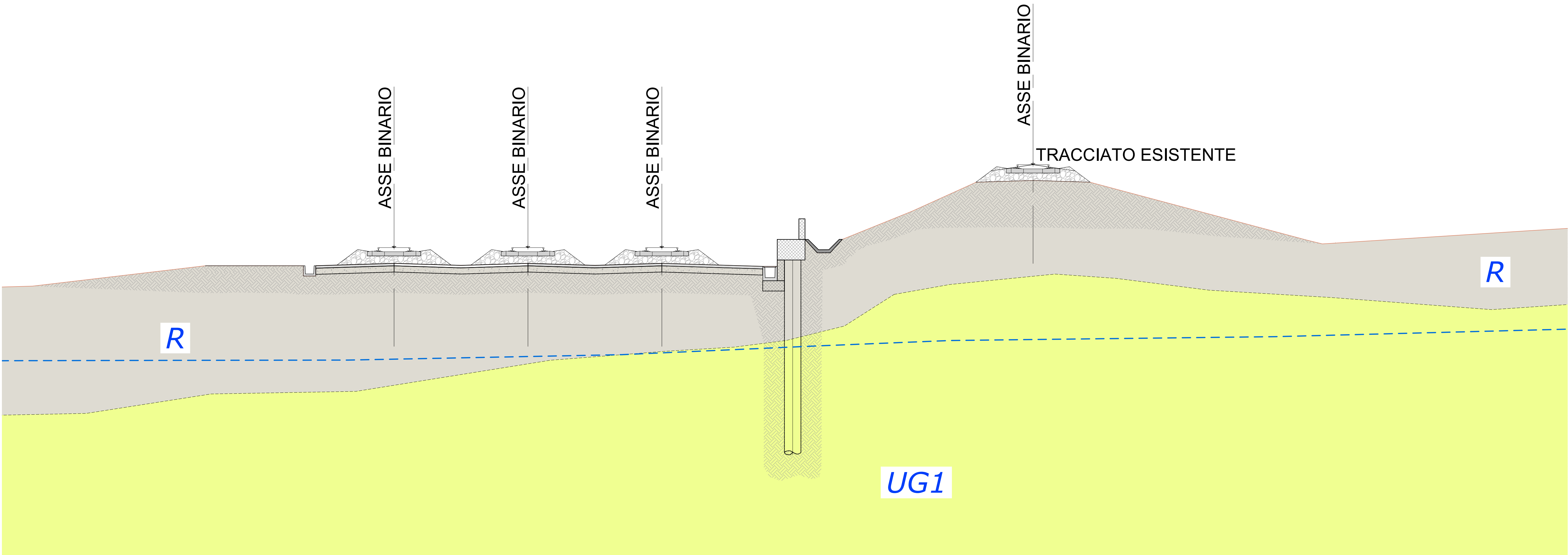
Sez km 0+500 (Fascio di Binari) Scala 1 : 100
