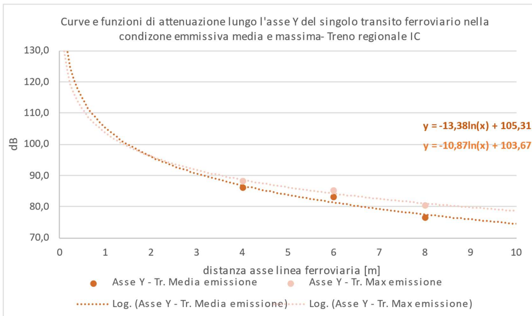
Figura 4-5 Linea ferroviaria all'aperto: curve e funzioni di attenuazione lungo l'asse Y del singolo evento transito associato ad un treno regionale IC nella condizione di emissione massima e media
