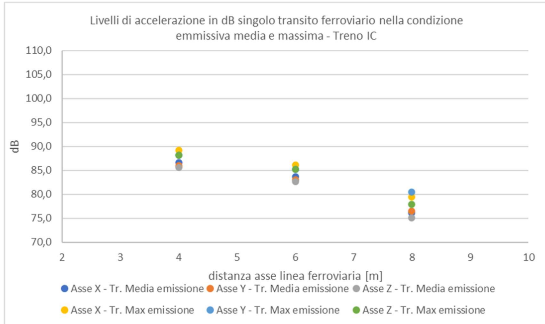
Figura 3-5 Postazione VIB_01, linea ferroviaria in rilevato: livelli di accelerazione rappresentativi delle condizioni di massima e media emissione di un singolo transito ferroviario a 4, 6 e 8 m dal binario più esterno - Treno Regionale IC
