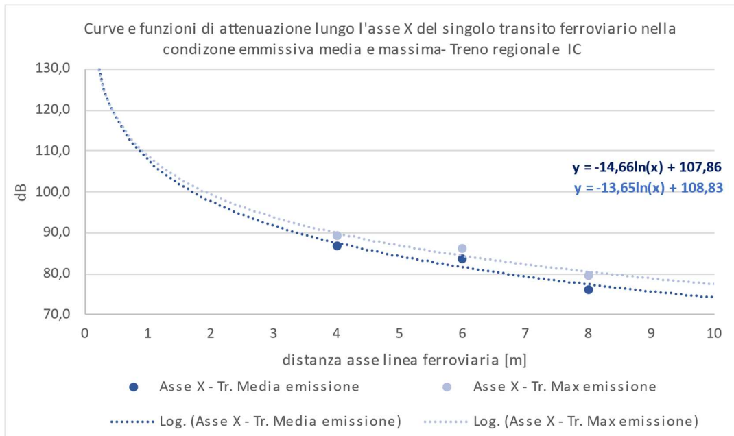
Figura 4-4 Linea ferroviaria all'aperto: curve e funzioni di attenuazione lungo l'asse X del singolo evento transito associato ad un treno regionale IC nella condizione di emissione massima e media
