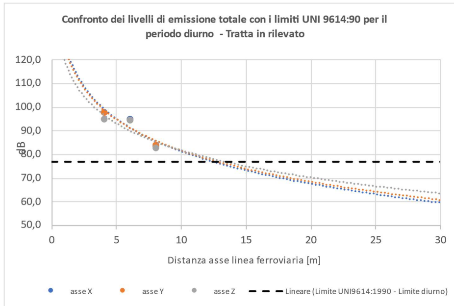
Figura 5-1 Confronto dei livelli di emissione complessiva all'interno degli edifici con i limiti UNI 9614:1990 in funzione della distanza dall'asse della linea secondo il modello di esercizio previsto – Tratta 1, sezione rilevato - Periodo diurno
