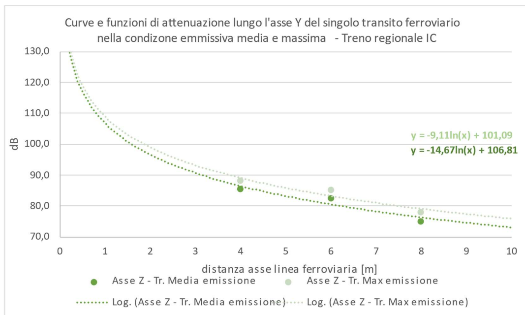
Figura 4-6 Linea ferroviaria all'aperto: curve e funzioni di attenuazione lungo l'asse Z del singolo evento transito associato ad un treno regionale IC nella condizione di emissione massima e media
