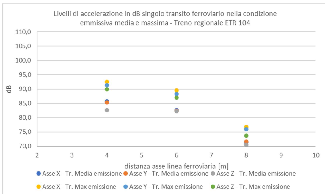
Figura 3-4 Postazione VIB_01, linea ferroviaria in rilevato: livelli di accelerazione rappresentativi delle condizioni di massima e media emissione di un singolo transito ferroviario a 4, 6 e 8 m dal binario più esterno - Treno Regionale ETR 104
