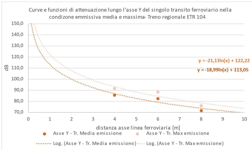
Figura 4-2 Linea ferroviaria all'aperto: curve e funzioni di attenuazione lungo l'asse Y del singolo evento transito associato ad un treno regionale ETR104 nella condizione di emissione massima e media
