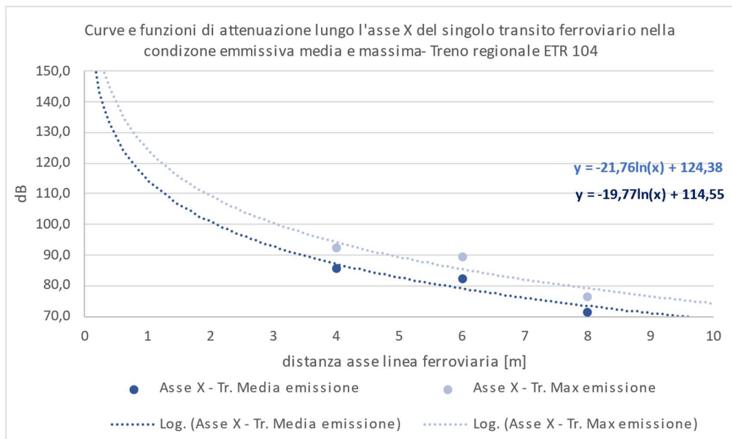
Figura 4-1 Linea ferroviaria all'aperto: curve e funzioni di attenuazione lungo l'asse X del singolo evento transito associato ad un treno regionale ETR104 nella condizione di emissione massima e media
