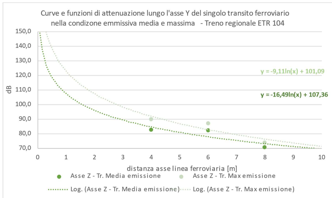
Figura 4-3 Linea ferroviaria all'aperto: curve e funzioni di attenuazione lungo l'asse Z del singolo evento transito associato ad un treno regionale ETR 104 nella condizione di emissione massima e media
