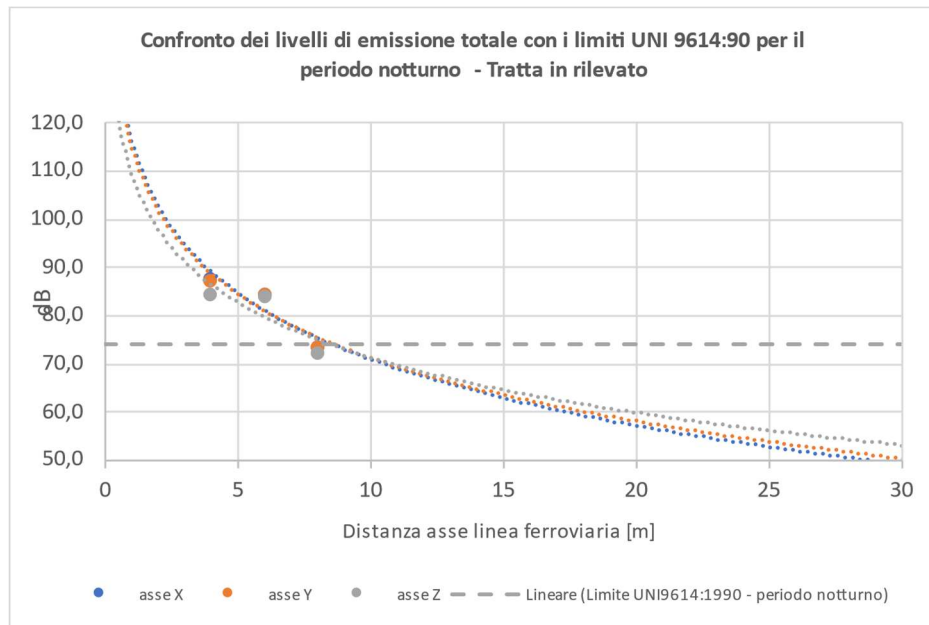
Figura 5-2 Confronto dei livelli di emissione complessiva all'interno degli edifici con i limiti UNI 9614:1990 in funzione della distanza dall'asse della linea secondo il modello di esercizio previsto – Tratta 1, sezione rilevato - Periodo notturno
