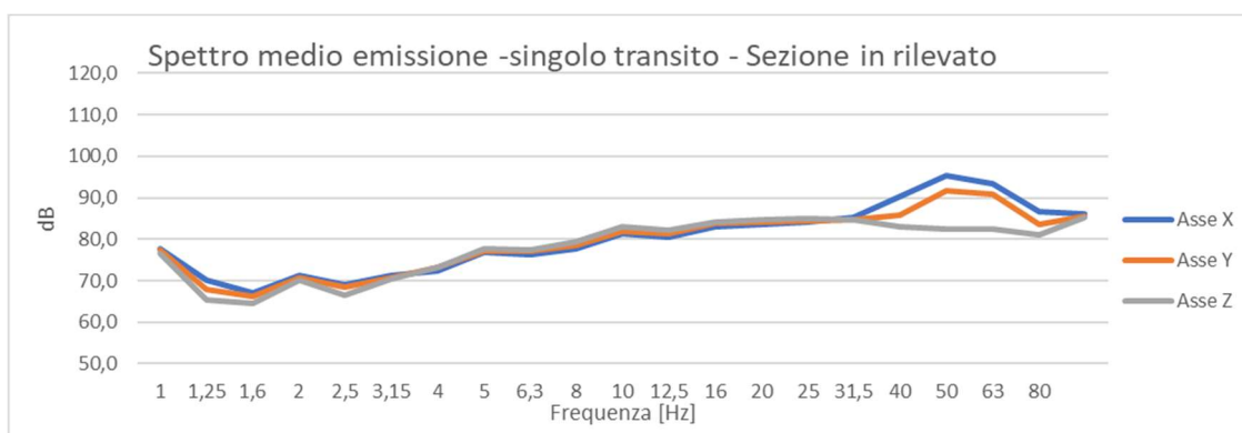
Figura 3-3 Spettro medio dei transiti rilevati presso la postazione T1 in prossimità del binario
