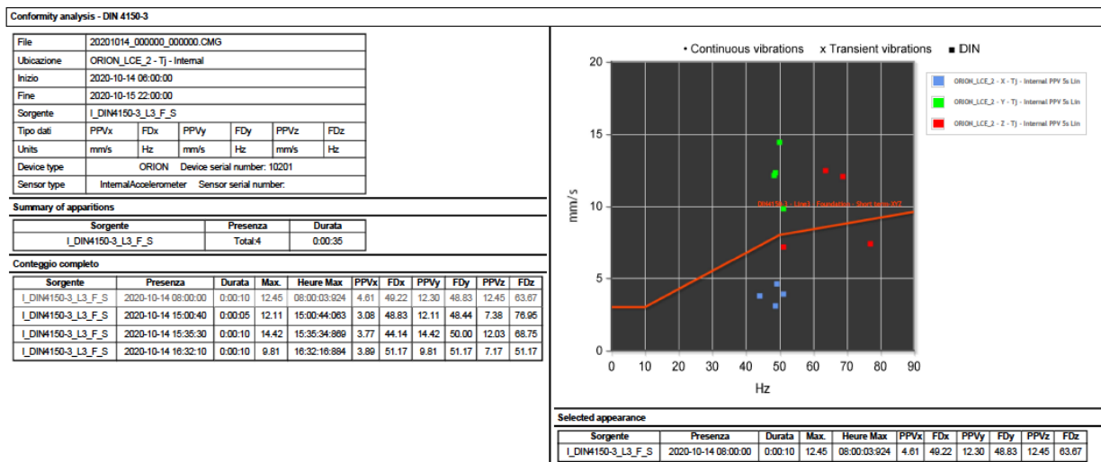
Esempio di resoconto analisi di vibrazioni
