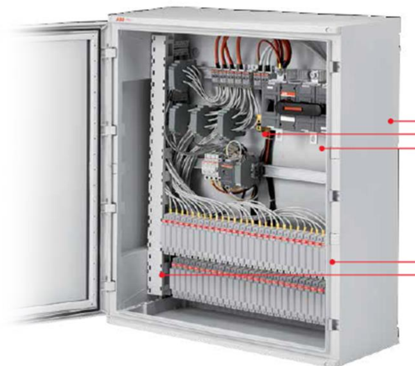
Figura 6.1.2.1 String box tipo
