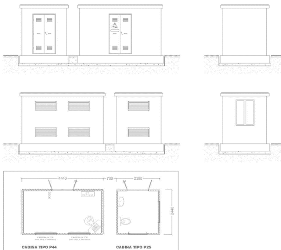
Figura 6.3.5.1 – locali guardiania e w.c.
