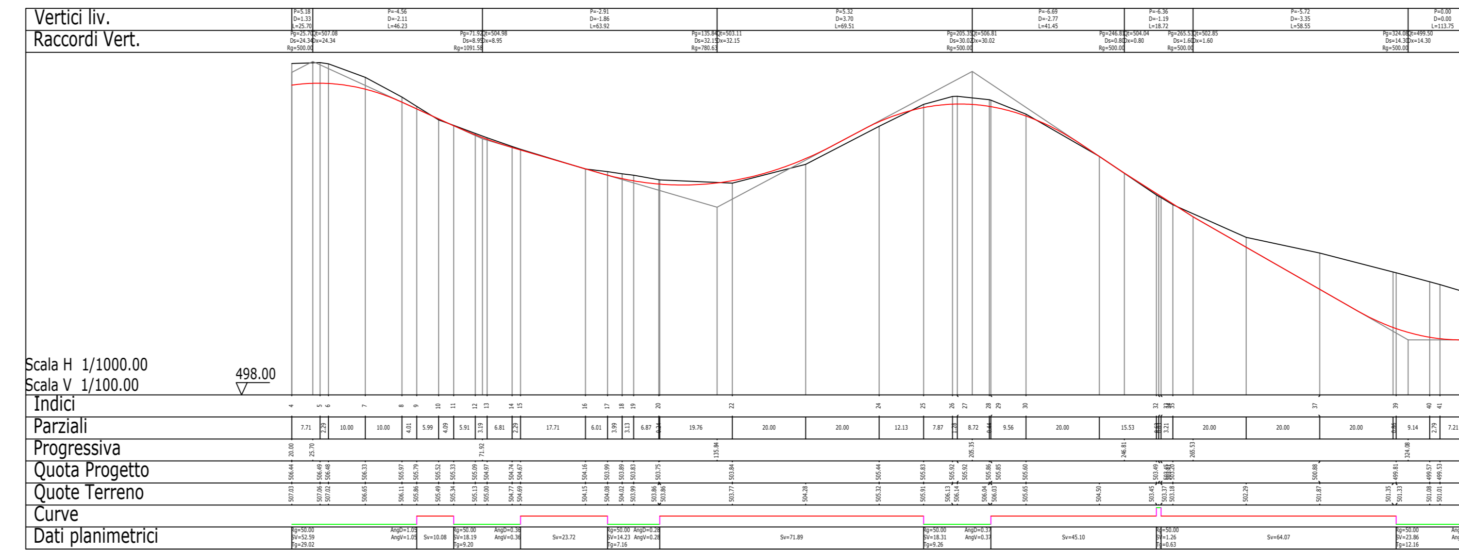
TRATTO 9-10 - VIABILITÀ DI IMPIANTO - POSTAZIONE AEROGENERATORE T05
