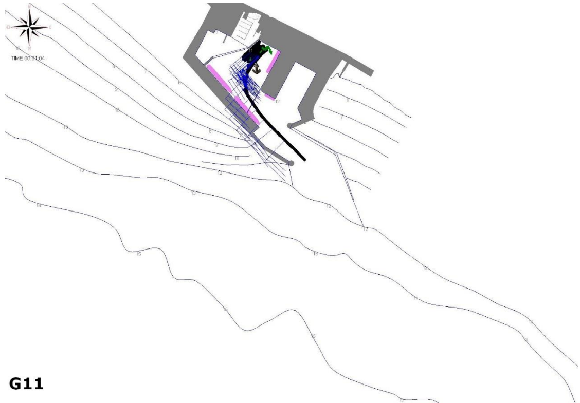
Fig. A - 37 – Manovra G11 – Ro-Ro 200 - Uscita - MANOVRA RIUSCITA Vento di Libeccio e onda – Intensità 25 nodi.
