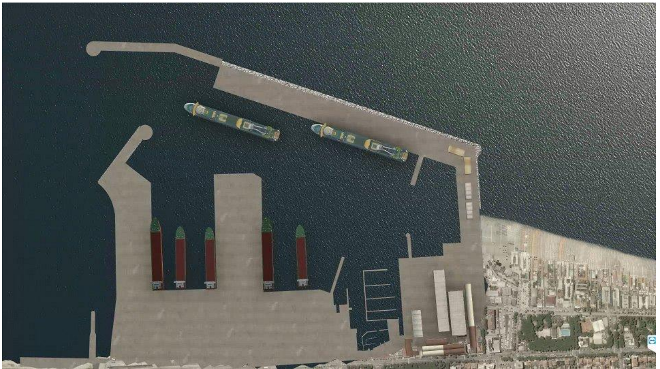
Fig. C - 2 – Vista 3D del layout di proposta di PRP utilizzato durante le simulazioni di manovra.
