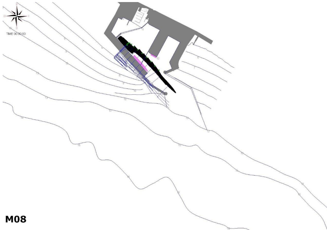
Fig. A - 8 – Manovra M08– Cruise 330 - Uscita - MANOVRA RIUSCITA Vento di Libeccio e onda - Intensità 25 nodi.
