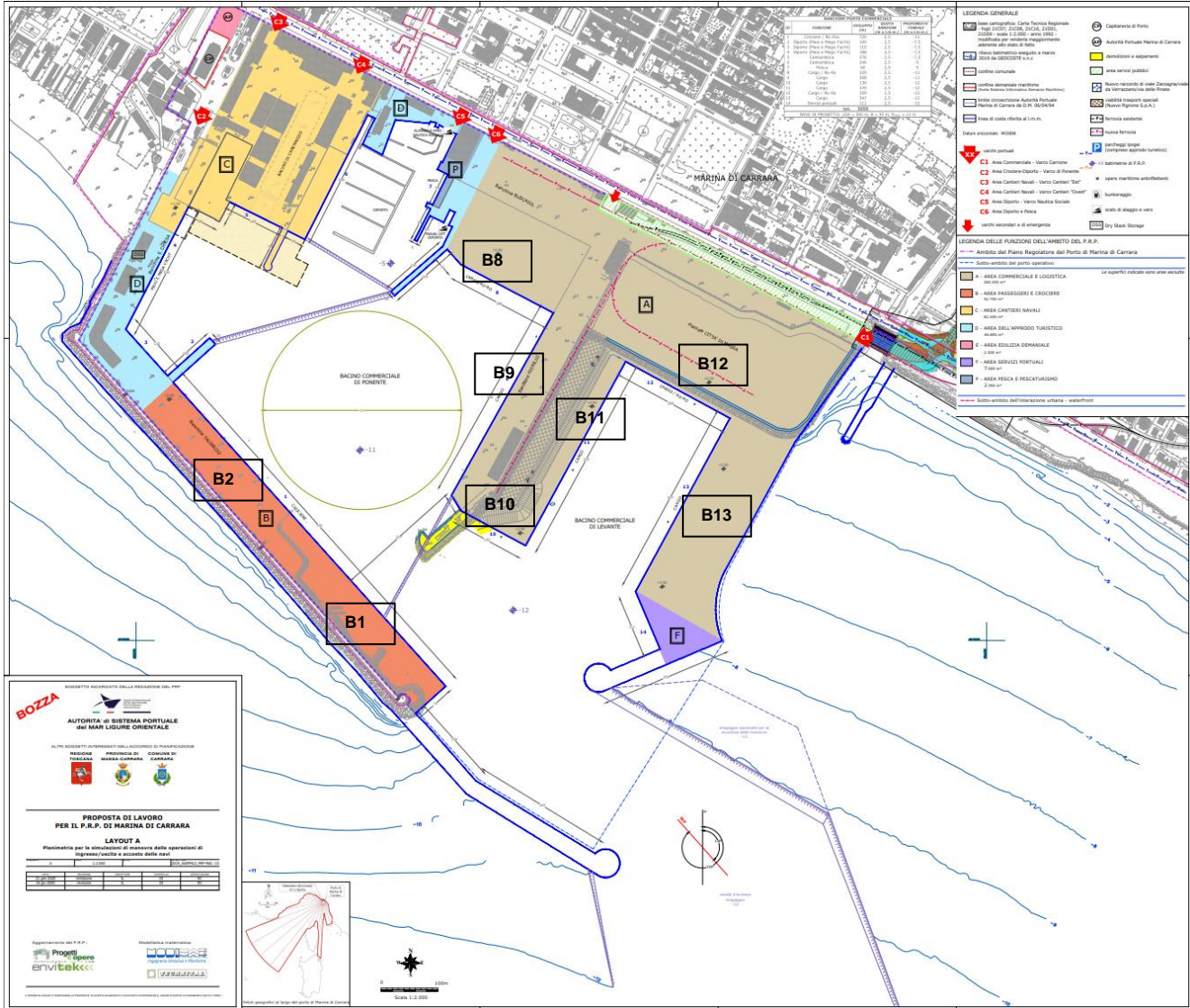
Fig. 23 Porto di Marina di Carrara – Layout di proposta di PRP
