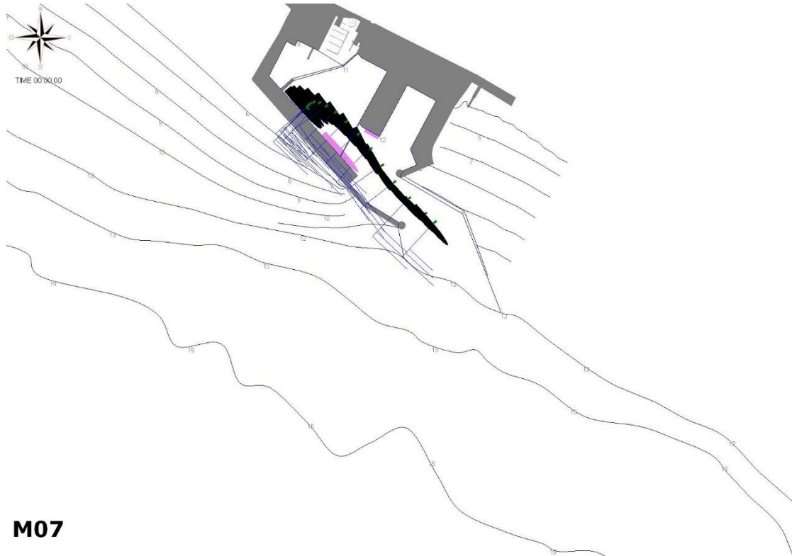
Fig. A - 7 – Manovra M07– Cruise 330 - Uscita - MANOVRA RIUSCITA Vento di Libeccio e onda - Intensità 25 nodi.
