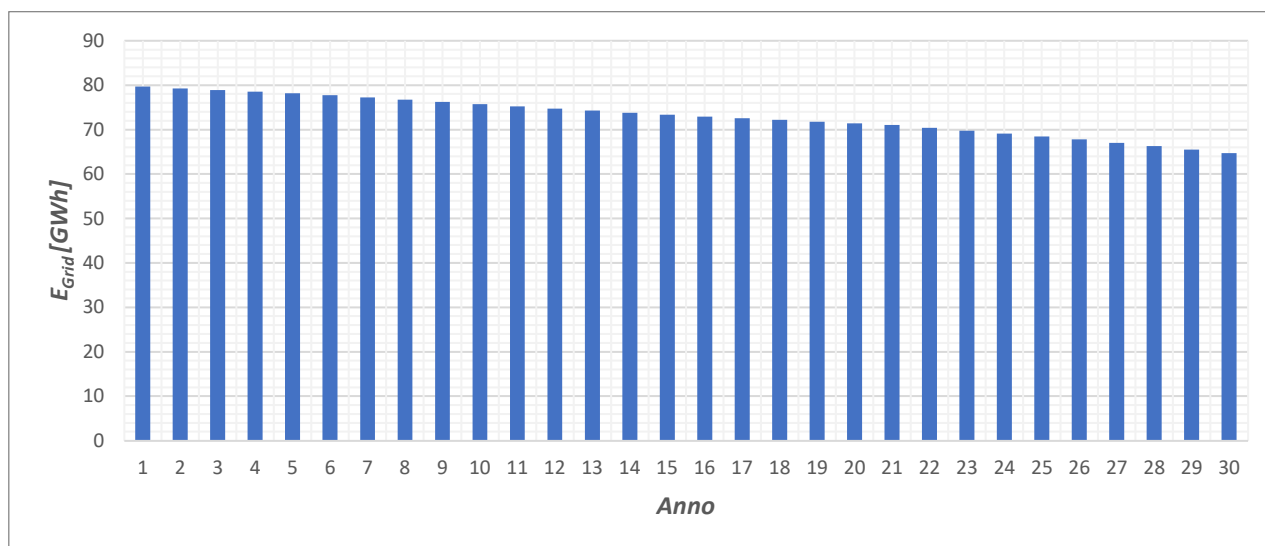
Figura 5 - Energia immessa in reta nei 30 anni di vita dell'impianto - Dati esportati dal software di calcolo PVSyst
