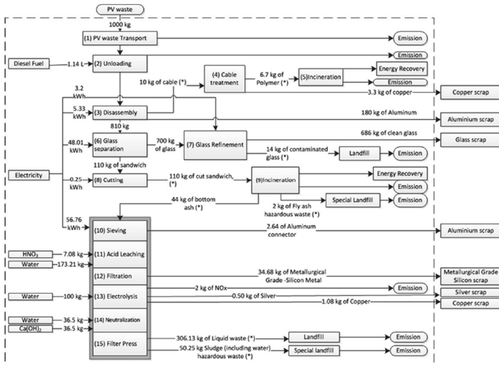
Figura 9 - Diagramma di flusso relativo al trattamento dei rifiuti da fotovoltaico (Latessa C.L. et al.2016a). 30
