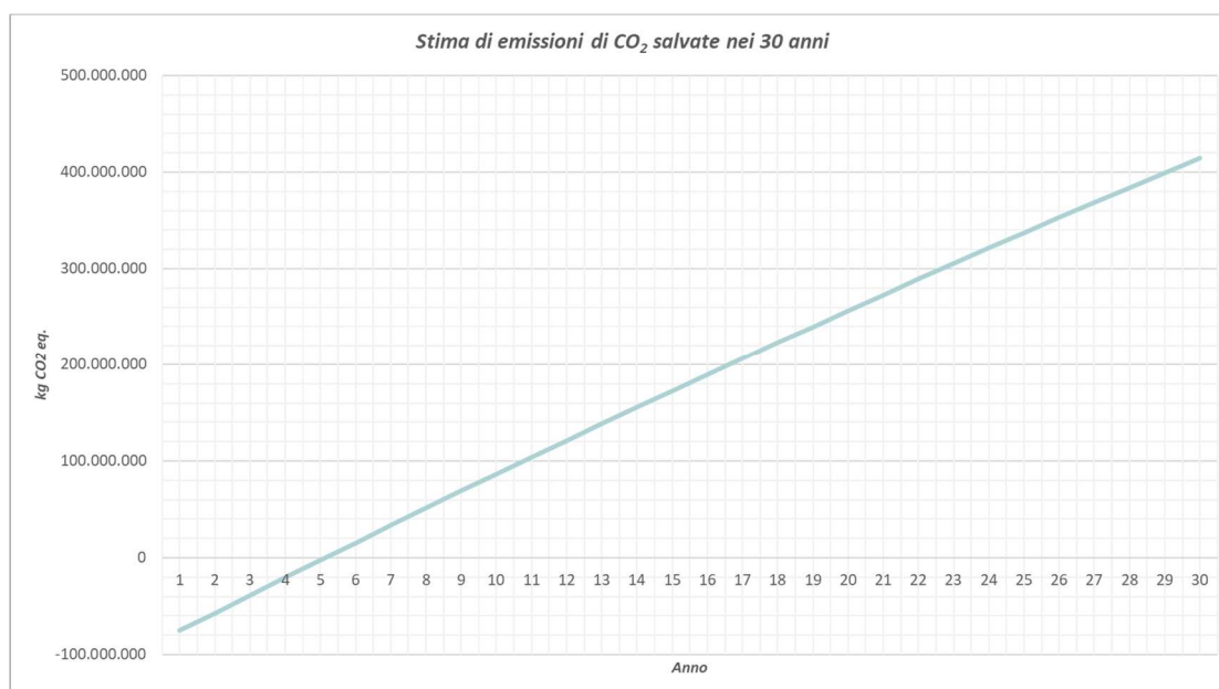
Figura 10 – Stima di risparmi di CO 2 nei 30 anni di vita dell'impianto fotovoltaico.
