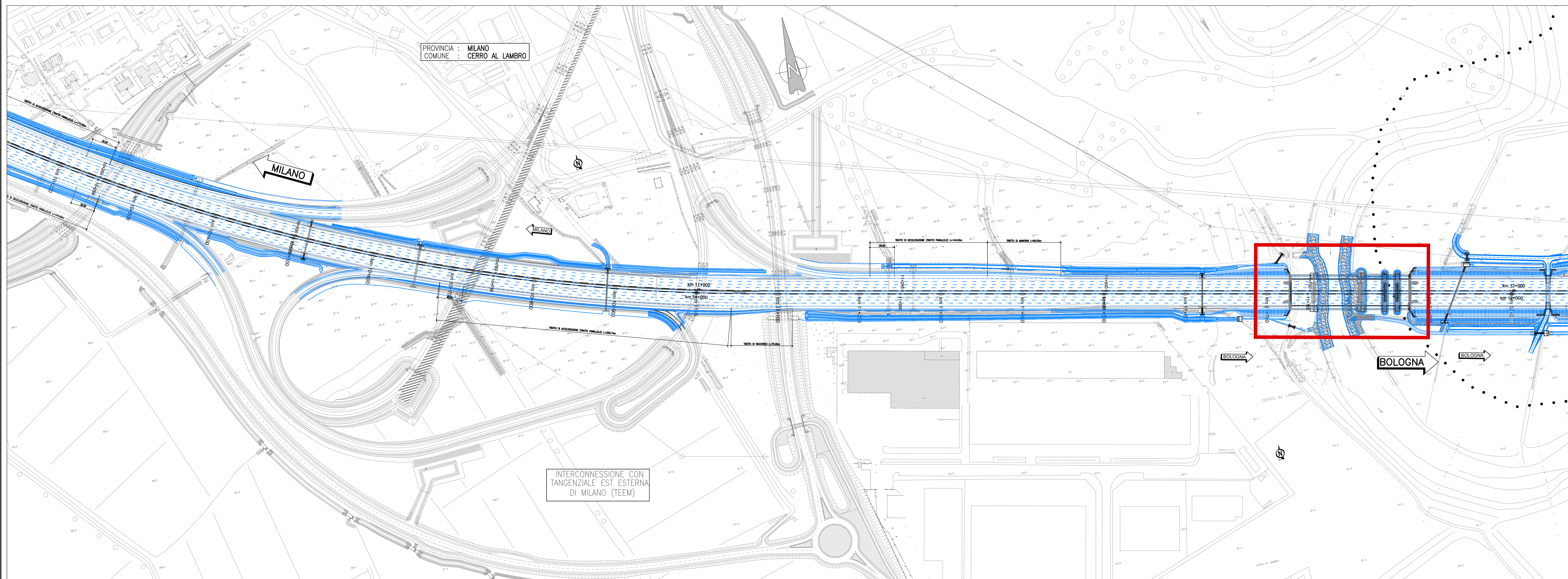
PLANIMETRIA DI PROGETTO (1:2.000)
