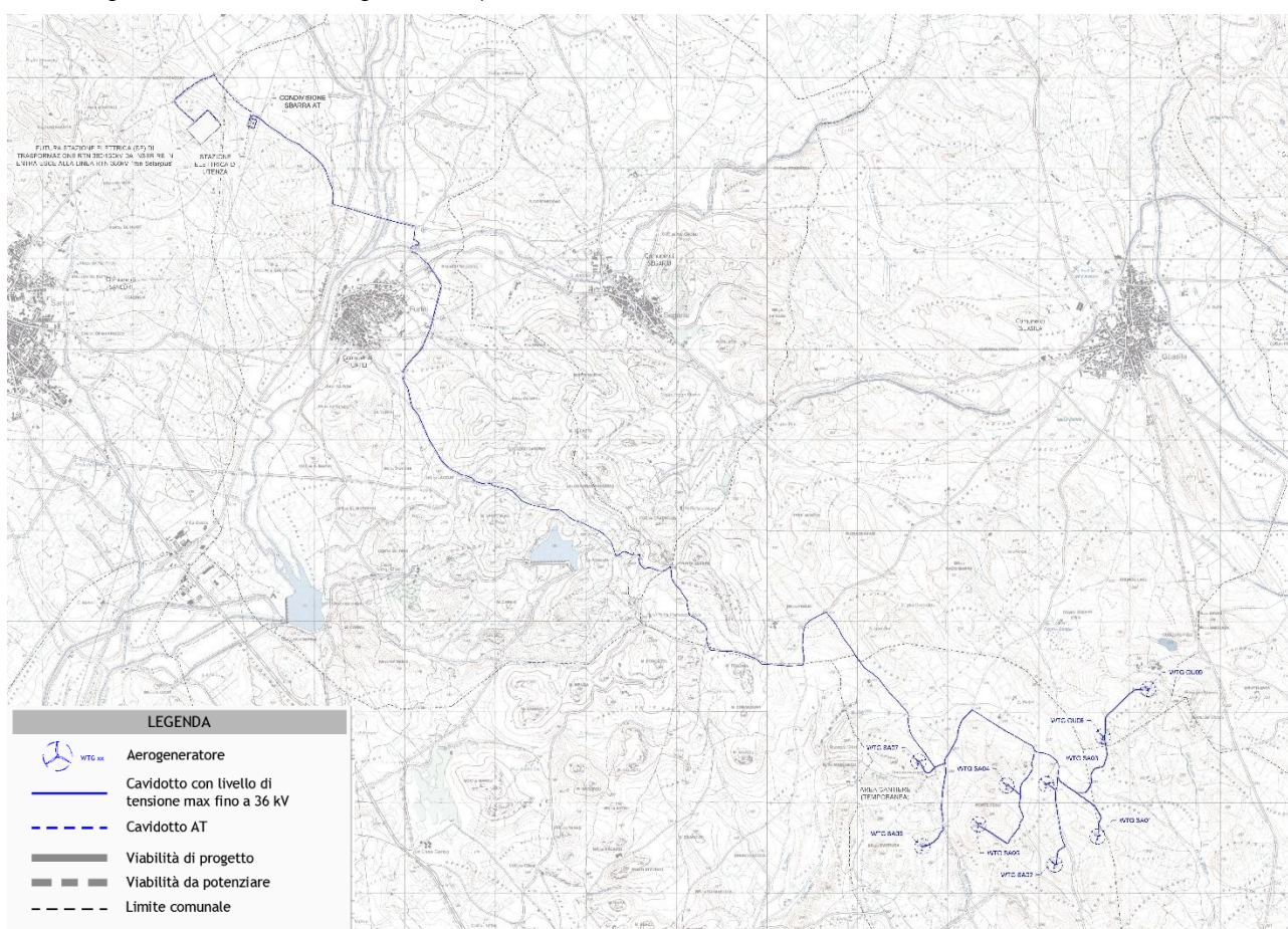
Figura 1 – Stralcio corografia d’inquadramento impianto di produzione energia rinnovabile da fonte eolica con annessi cavidotto, stazione elettrica di utenza e impianto di utenza per la connessione
