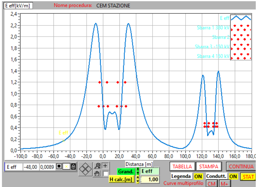
Campo elettrico lungo la sezione A-A, generato dalle 4 sbarre, sempre inferiore a 2.5 kV/m.
