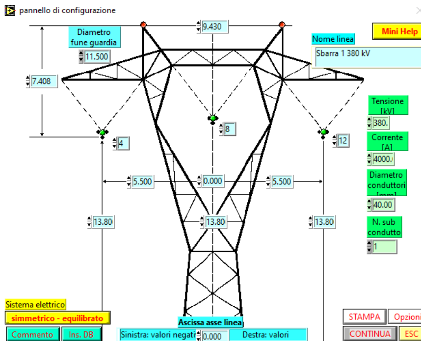
Configurazione geometrica sbarra 1.
