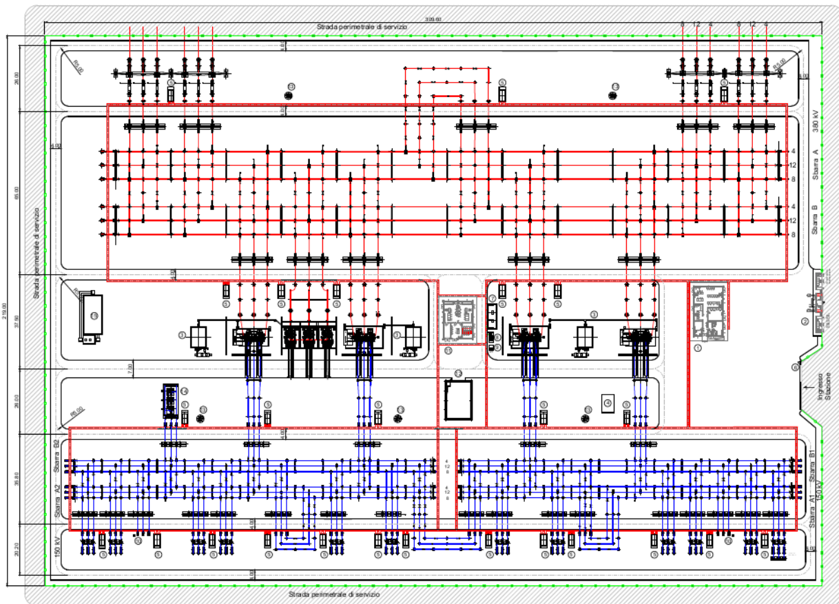
Planimetria SE Sanluri
