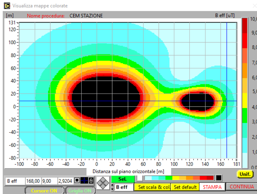
Campo elettromagnetico generato dalle 4 sbarre con verso della corrente concorde.
