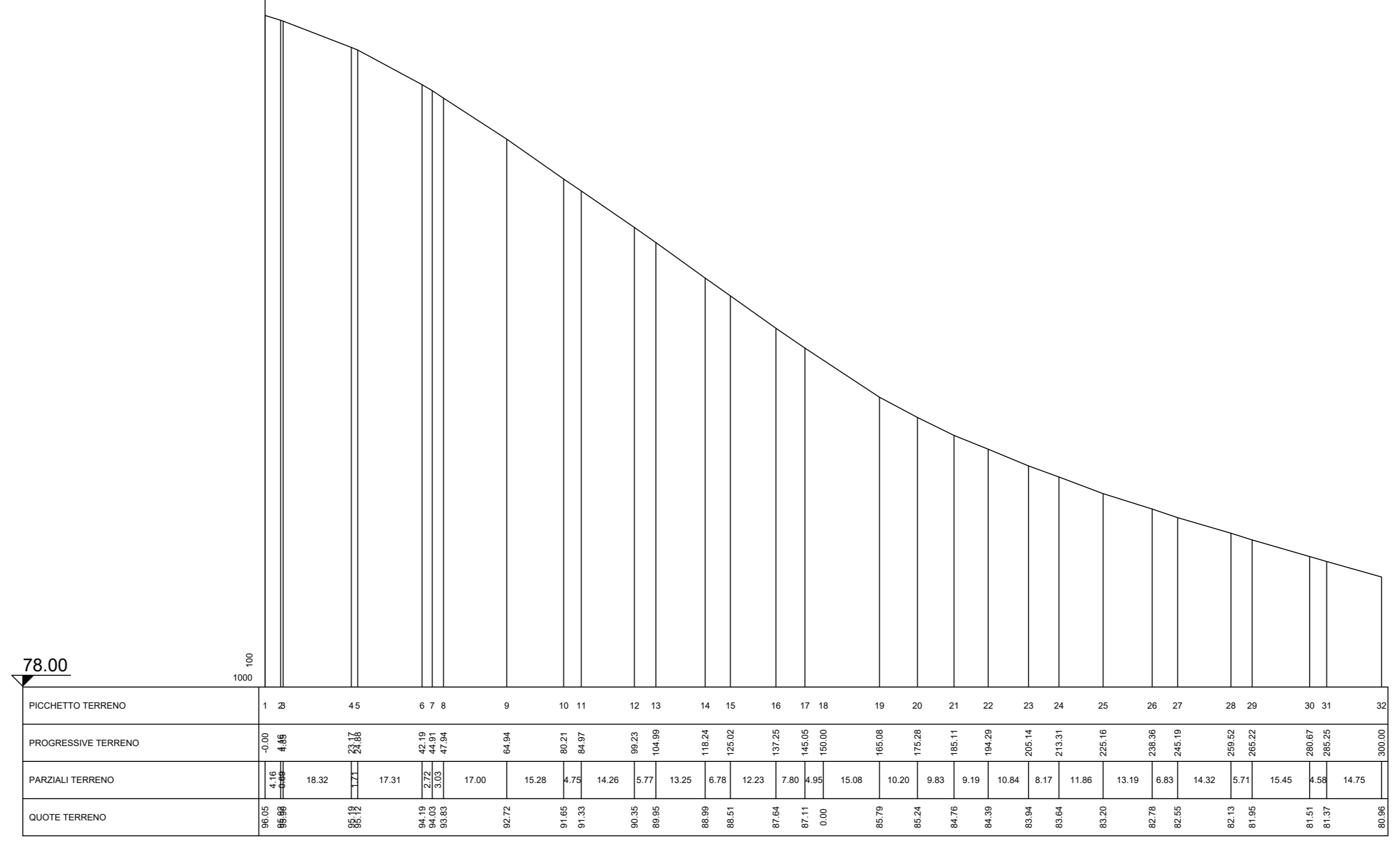
Sezione: TT' Progressiva: 0.00
