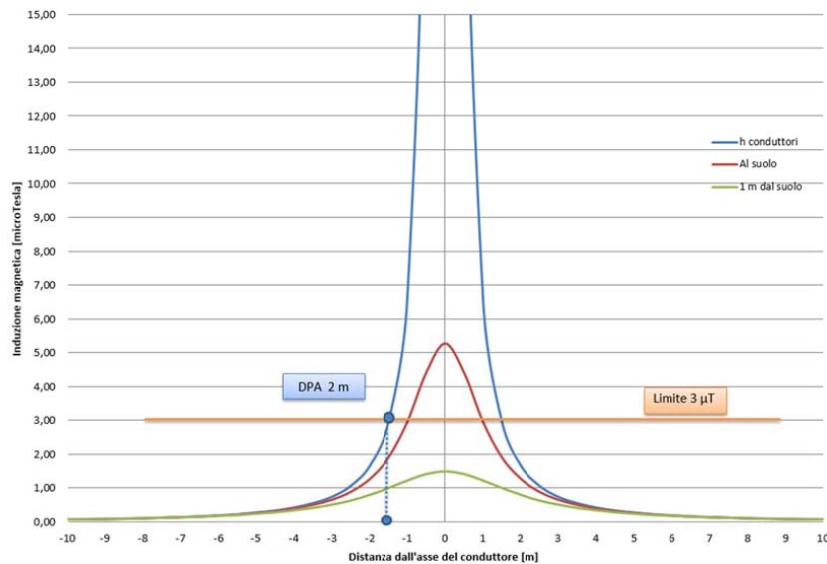
Figura 6 : Andamento del campo magnetico in funzione della distanza dall'asse dei conduttori relativa alla simulazione S2
