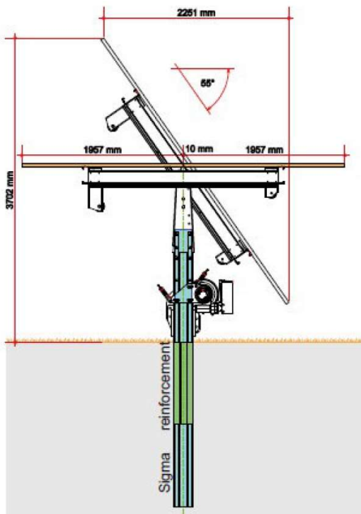
FIGURA 4 - TRACKER SOLARE TIPO
