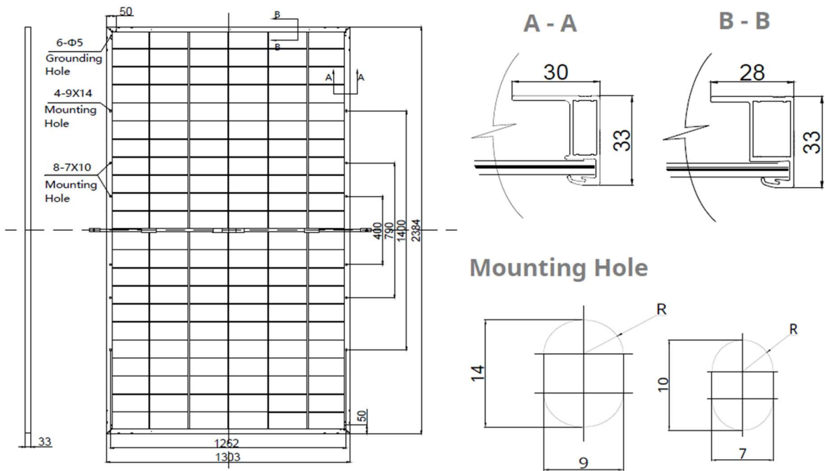
Figura 1: pannello FV fino a 580 Wp con dimensioni 2384 x 1303 x 33 mm
