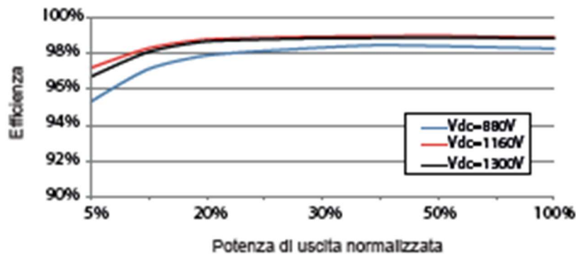
Figura 5: Caratteristiche salienti dell'inverter da 339 KW scelto
