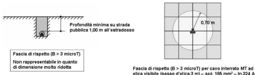
Figura 1: schema linee di cavo interrato
