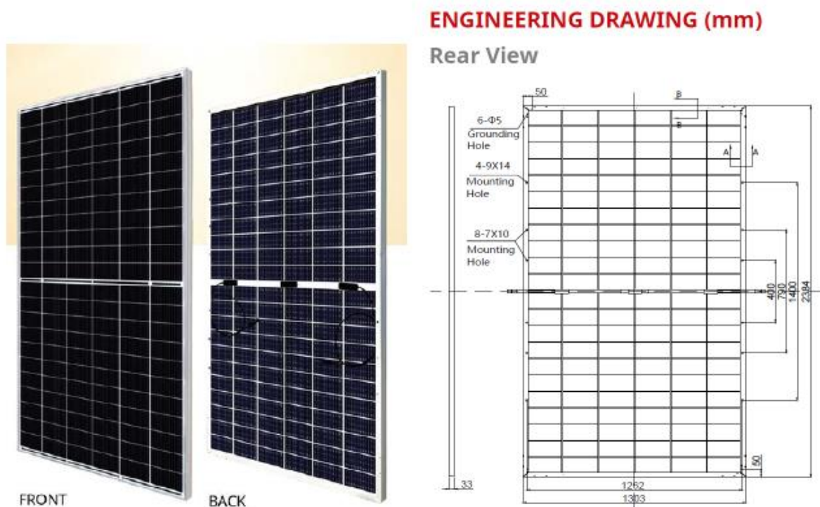
Figura 62. Pannello FV fino a 665 Wp con dimensioni 2384 x 1303 x 35 mm esempio
