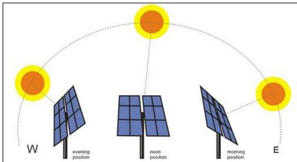
Figura 63. Variazione della posizione del tracker e dunque del modulo in funzione delle ore del giorno
