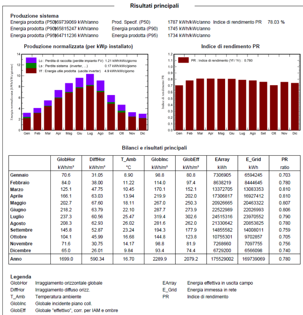
Figura 68. Dati meteorologici e risultati principali simulazione con PVSyst
