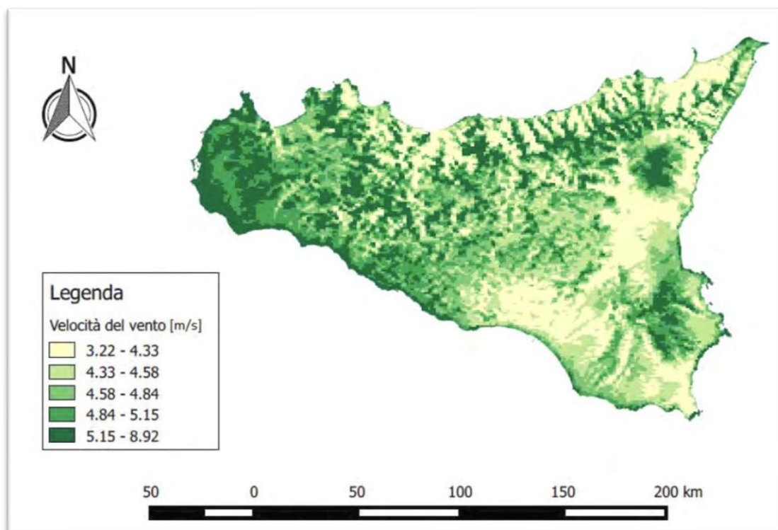
Figura 74. Velocità media del vento a 25 metri dal suolo (anni '70 - 2006) - Fonte: Atlante Eolico - GSE
