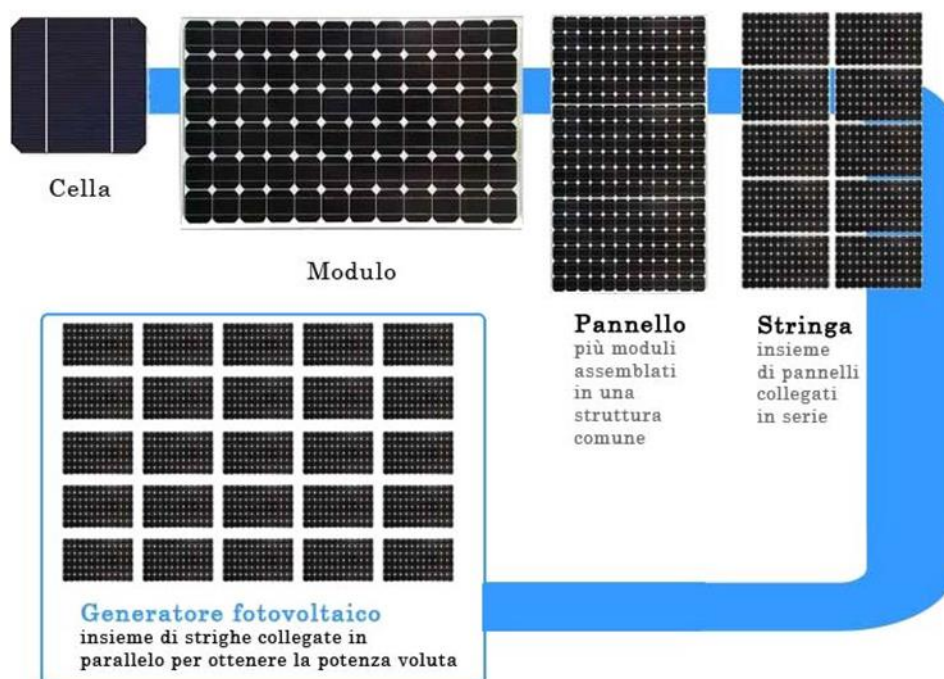
Figura 61. Unità elementari del generatore fotovoltaico
