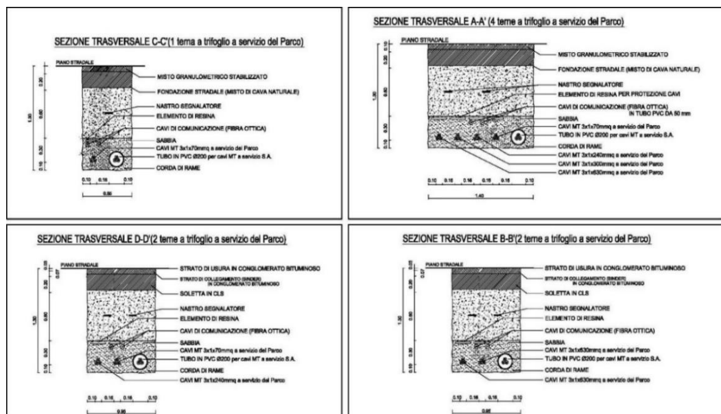
Figura 67. Differenti tipologie di posa del cavidotto
