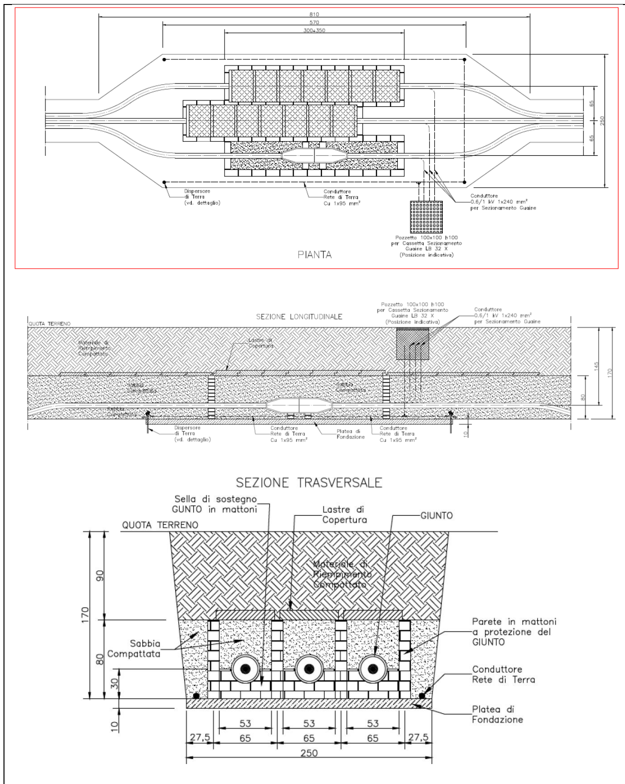
FIGURA 8: PIANTA E SEZIONI DEL TIPICO CAMERA DI GIUNZIONE
