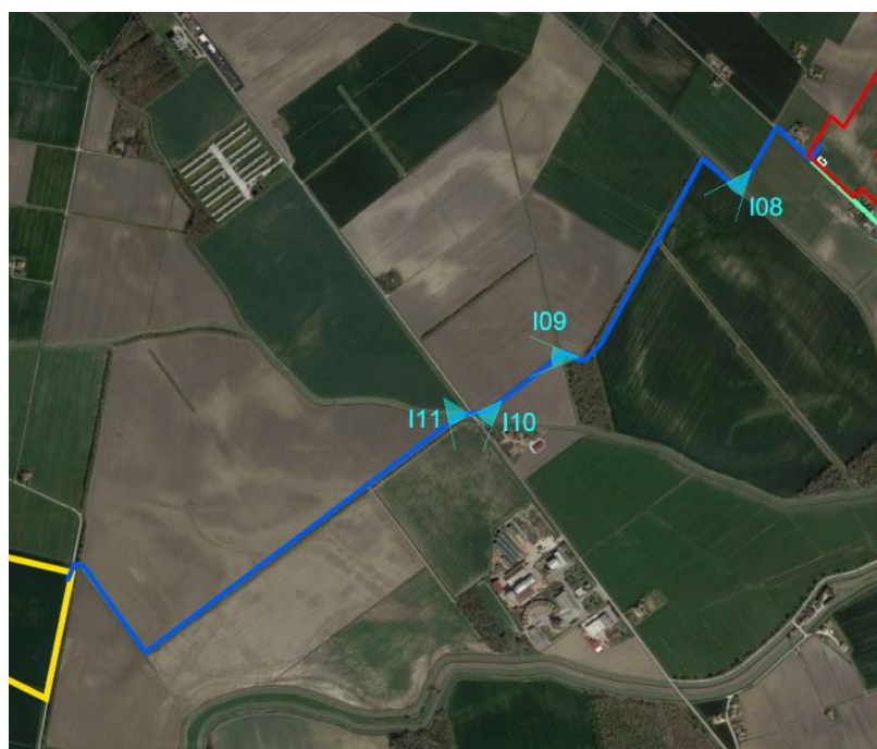
FIGURA 10: IDENTIFICAZIONE DELLE INTERFERENZE RILEVATE - PRIMO TRATTO
