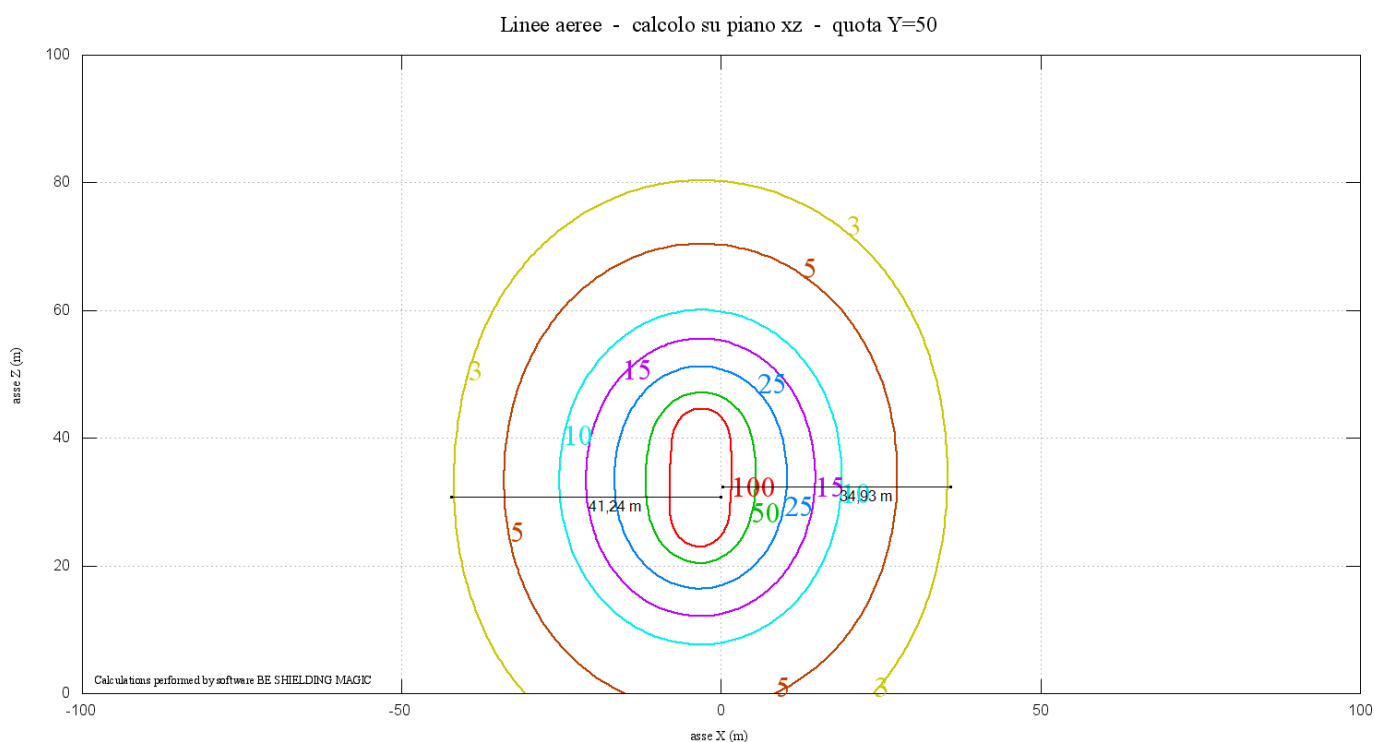
Figura 5 – Livelli di campo magnetico generato dai conduttori come disposti sul sostegno con mensola a bandiera
