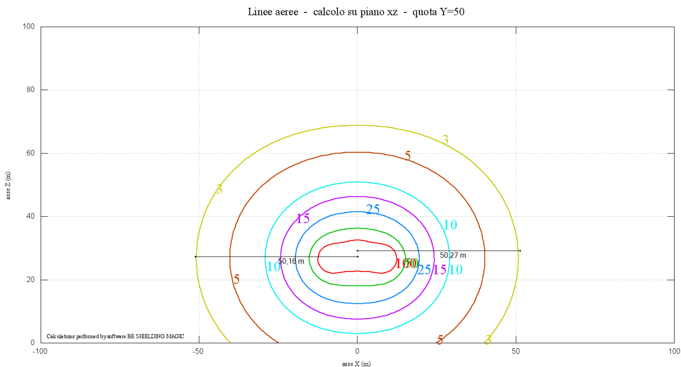
Figura 4 – Livelli di campo magnetico prodotti dalla configurazione dei conduttori su sostegno a Y con angolo
