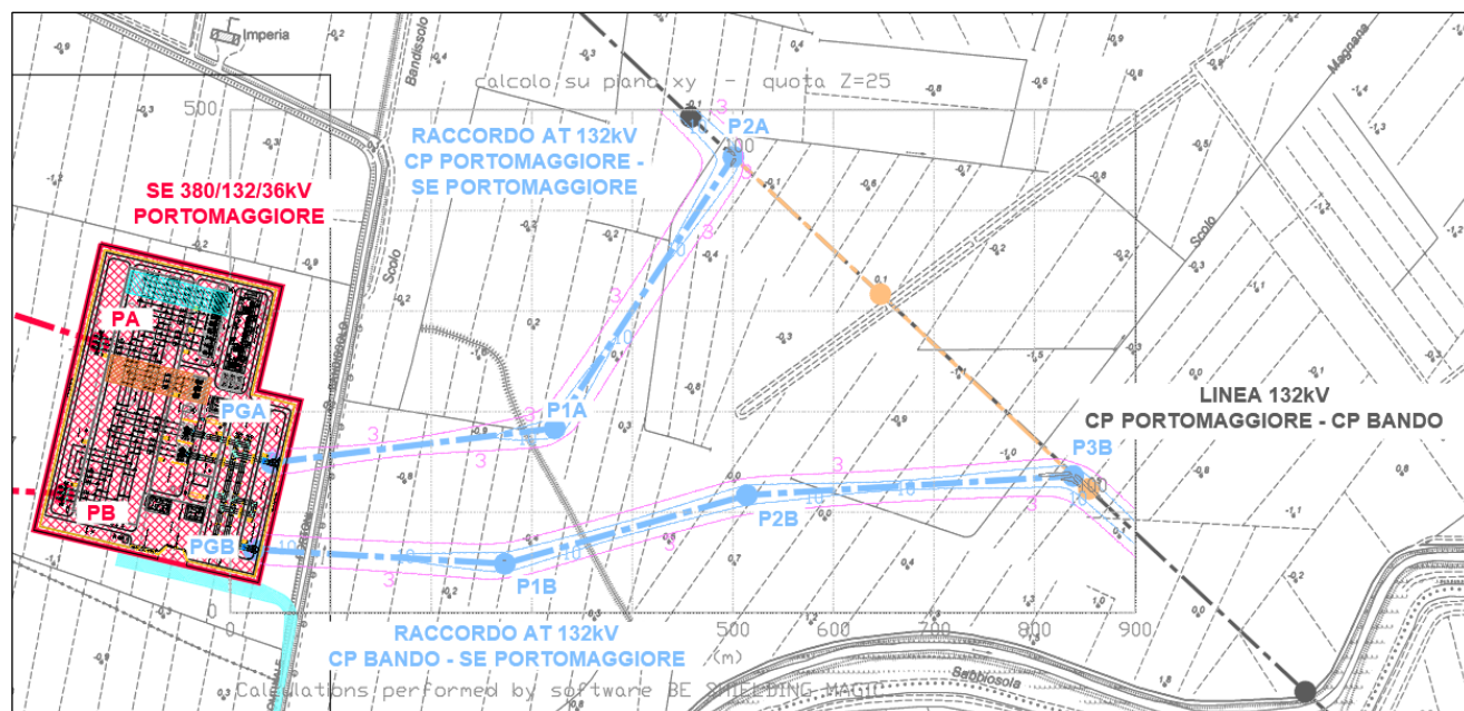
Figura 6 – Livelli di campo magnetico generato dai raccordi a 132 kV a 25 mslm
