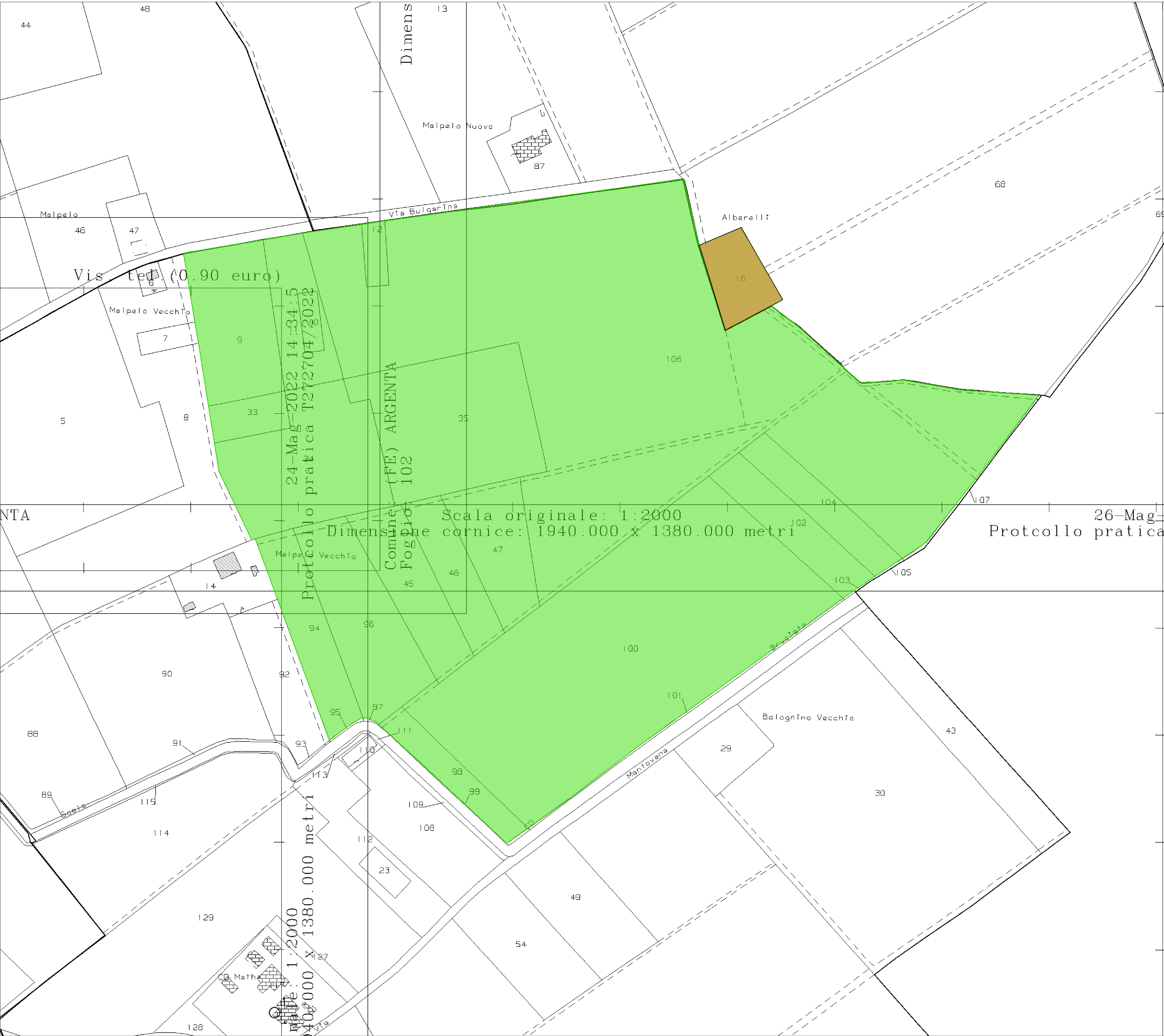
LAYOUT IMPIANTO - PIANO PARTICELLARE Scala 1:2000
