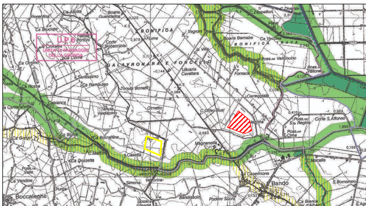
Figura 16: Tavola 5.7 Sistema Ambientale comune di Portomaggiore UdP 6 “della Gronda” (Fonte: PTCP Ferrara) – localizzazione impianto fotovoltaico (in rosso) e della stazione elettrica (in giallo)
