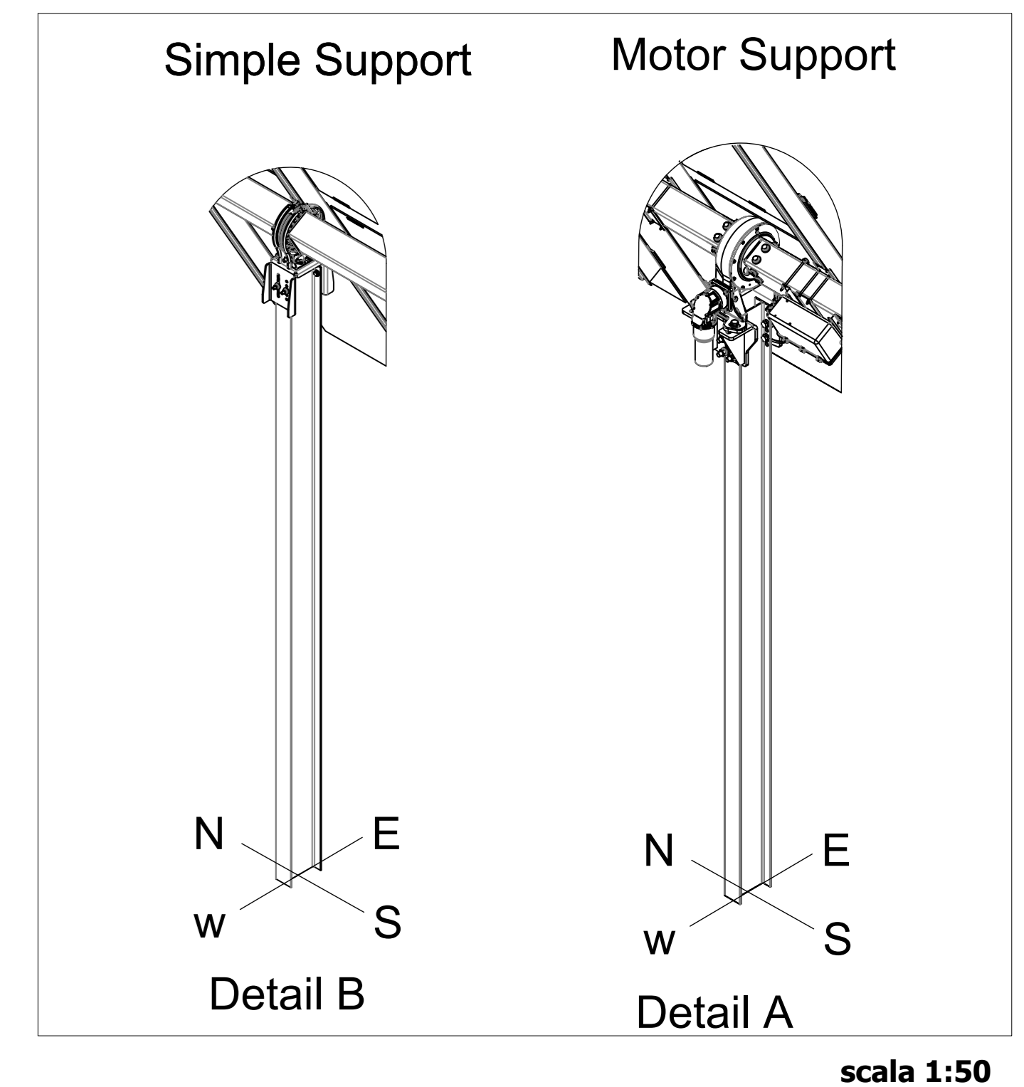
scala 1:50
