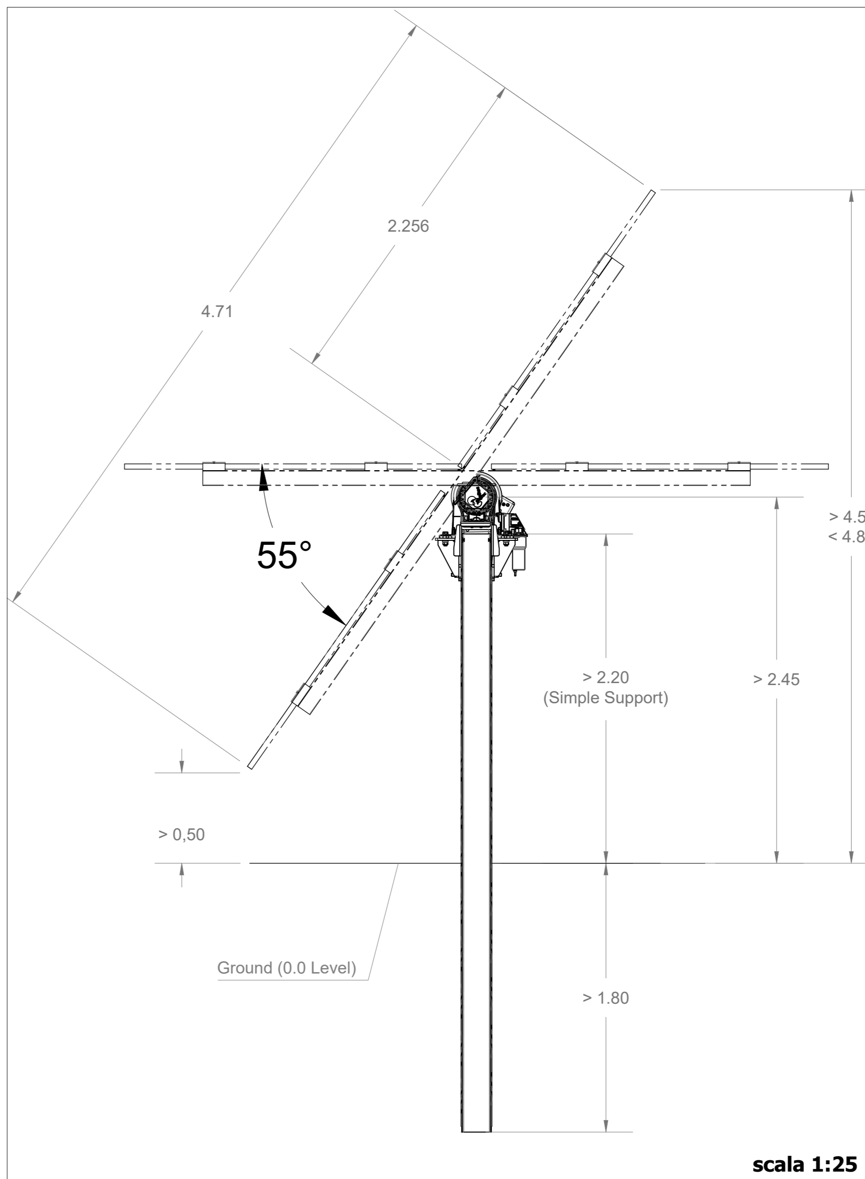
scala 1:25
