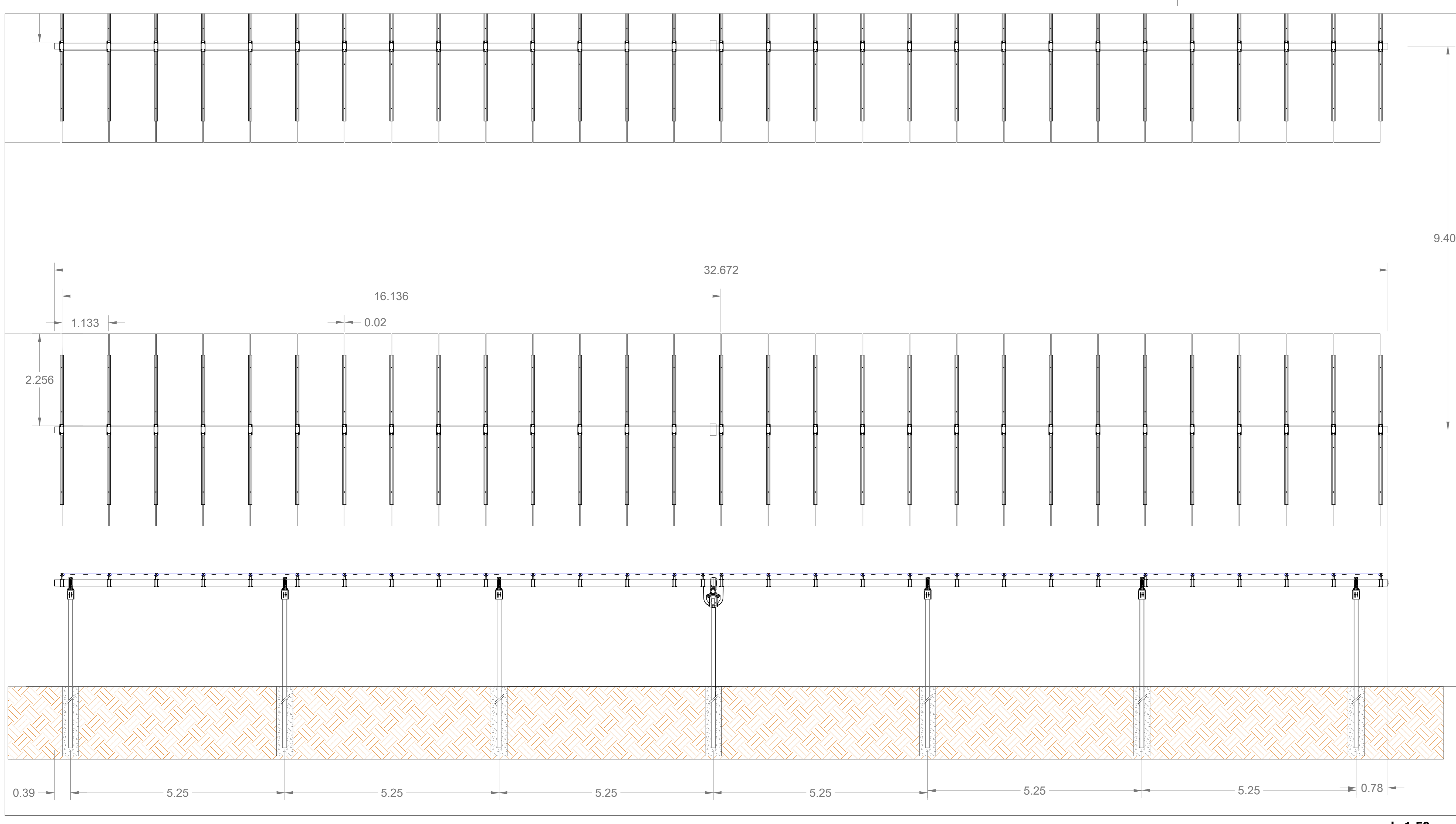
scala 1:50
