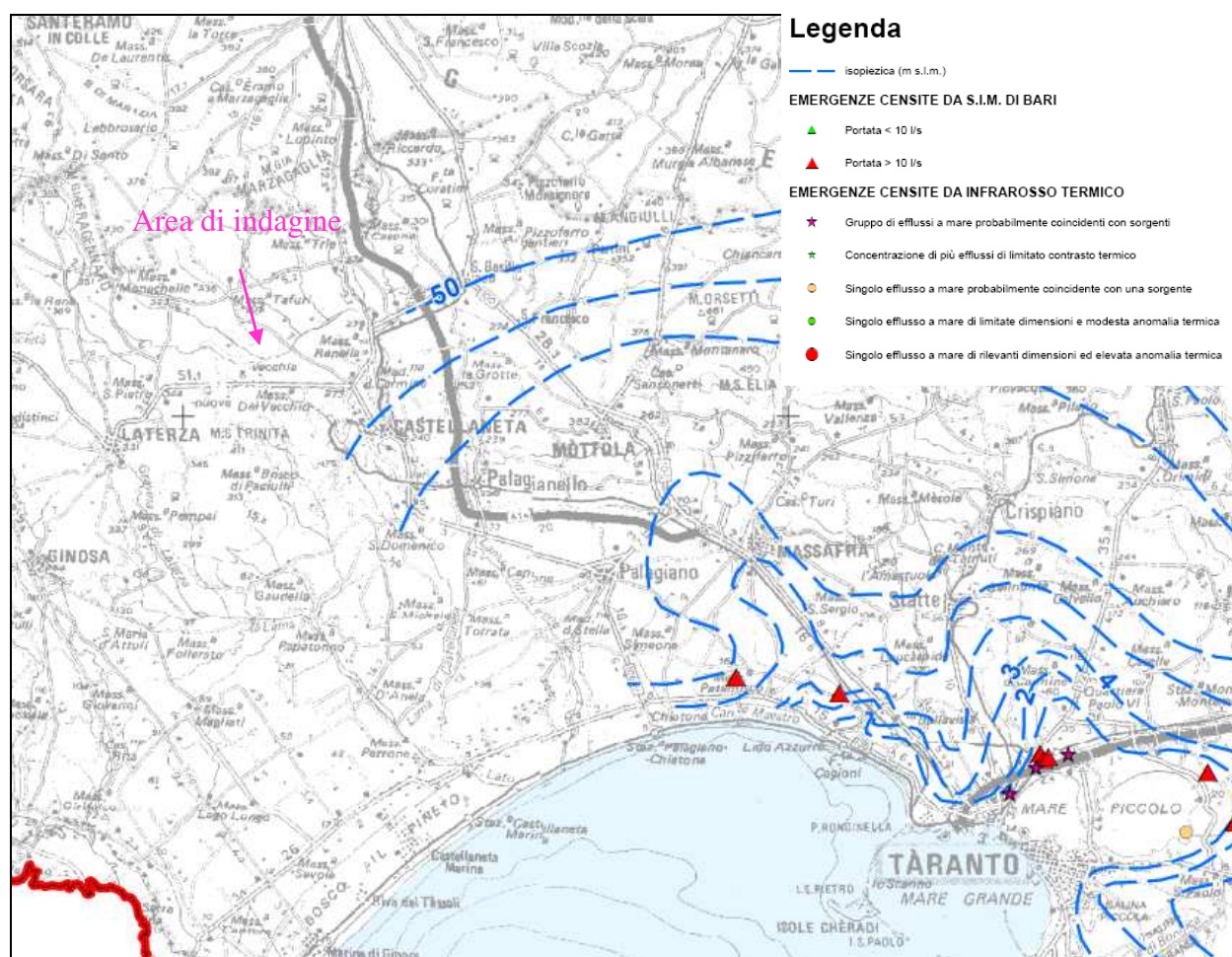
Fig. 1: Stralcio della carta della distribuzione media dei carichi piezometrici degli acquiferi carsici della Murgia e del Salento
