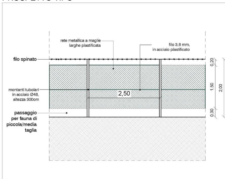
PROSPETTO TIPO
