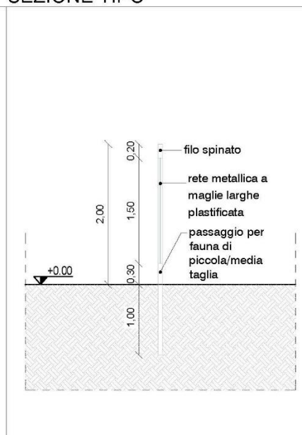
SEZIONE TIPO
