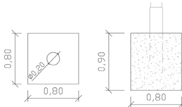
Figura 7 - Particolare costruttivo dello scavo dei pali di illuminazione e videosorveglianza
