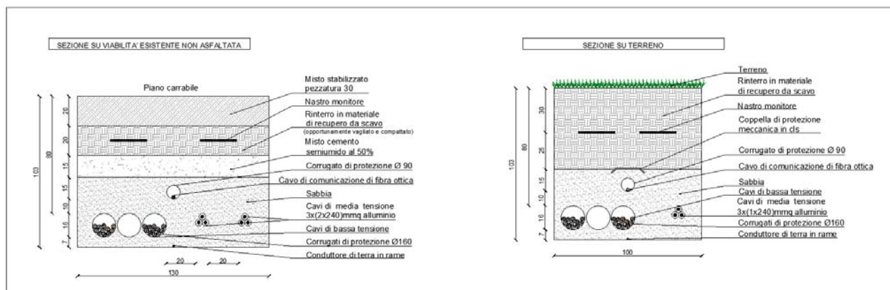
Figura 5 - Sezione tipo scavo trincea cavidotta BT-MT su strada non asfaltata (2 terne) e su terreno agricolo (1 terna)
