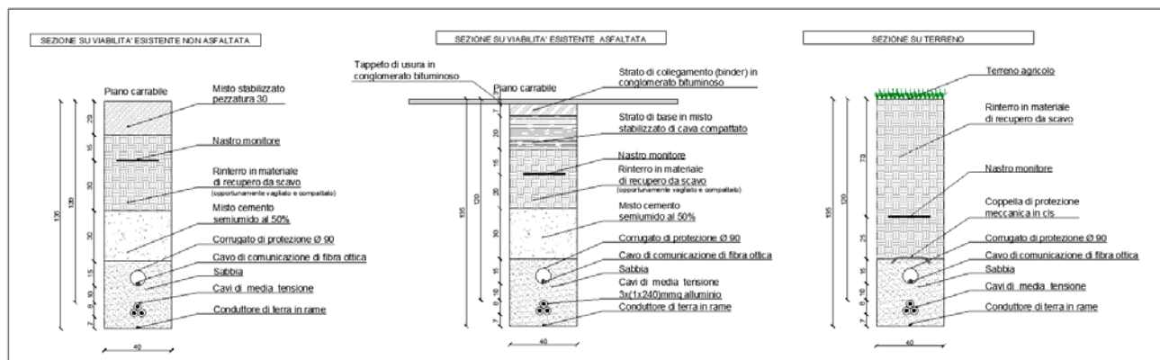
Figura 4 - Sezione tipo scavo trincea cavidotto MT (1 terna)
