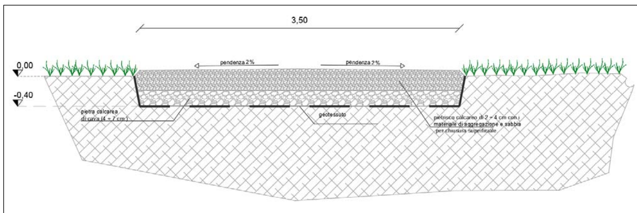
Figura 6 - Sezione tipo viabilità interna
