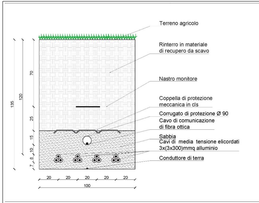
Figura 3 - Particolare sezione cavidotto esterno MT su terreno agricolo
