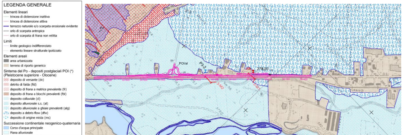
Figura 9: Stralcio della Carta Geologica di PD della tratta 3 - SS38
