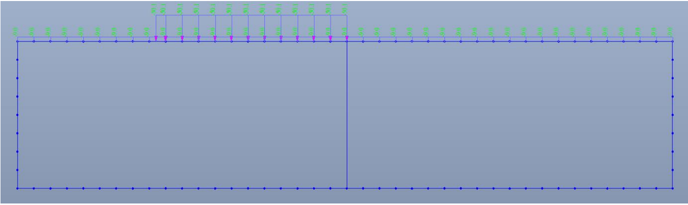
Figura 23: Sovraccarichi verticale da traffico con TS all'appoggio interno [kN/m]
