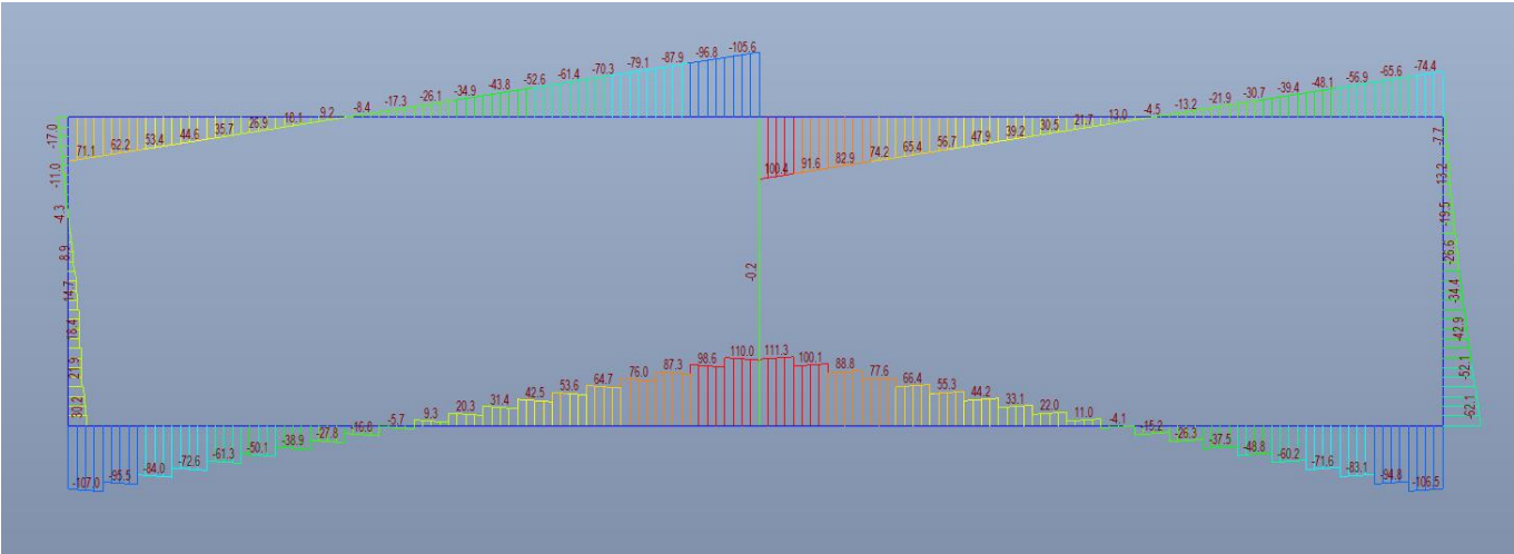
Figura 39: Involuppo SLV Taglio [kN]
