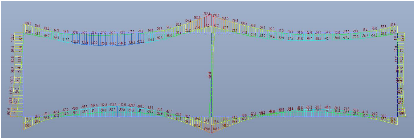
Figura 44: Involuppo SLE frequente Momento flettente [kNm]
