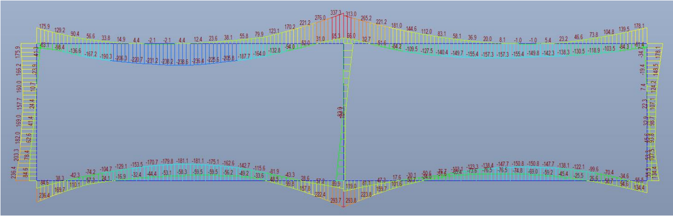
Figura 37: Involuppo SLU Momento flettente [kNm]
