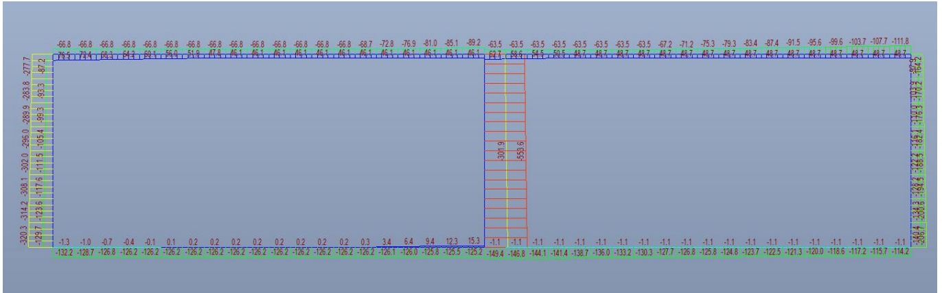
Figura 35: Involuppo SLU Azione assiale [kN]
