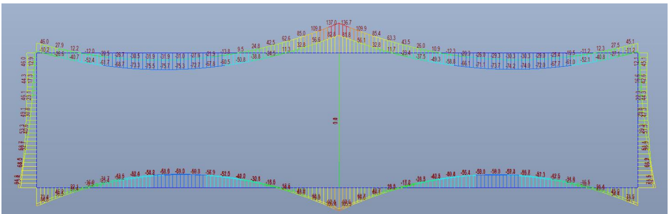
Figura 46: Involuppo SLE quasi permanente Momento flettente [kNm]
