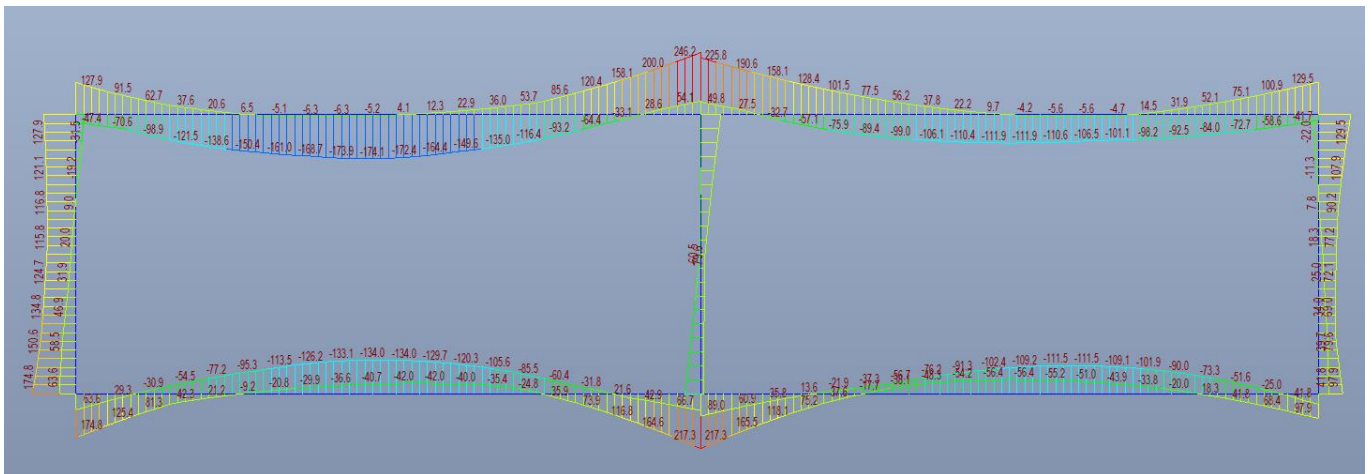
Figura 42: Involuppo SLE rara Momento flettente [kNm]
