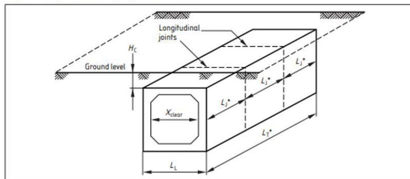
Figura 27: Azione di frenatura sullo scatolare
