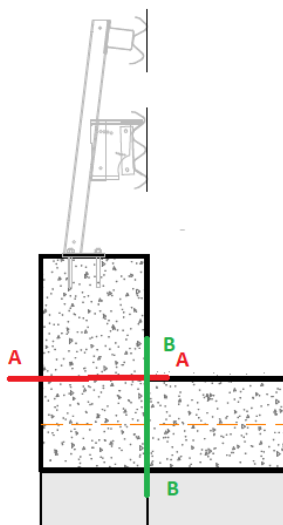
Figura 55: Sezioni di verifica ad urto
