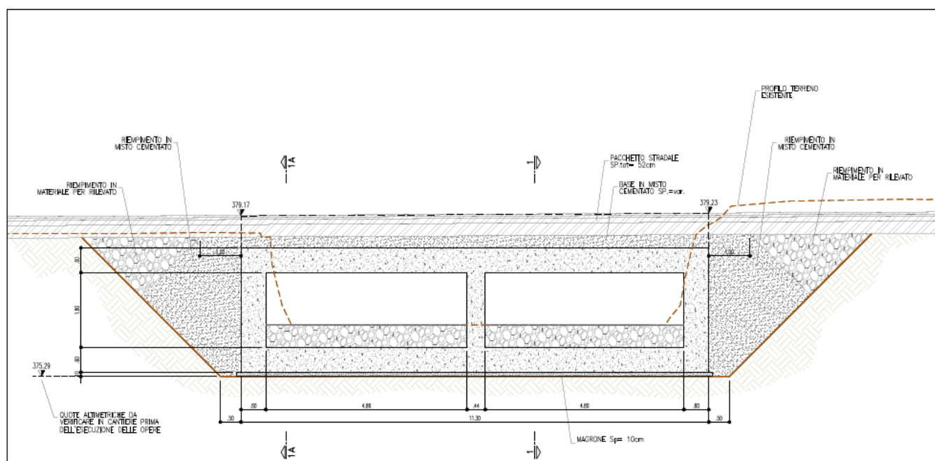
Figura 5: Sezione trasversale del tombino
