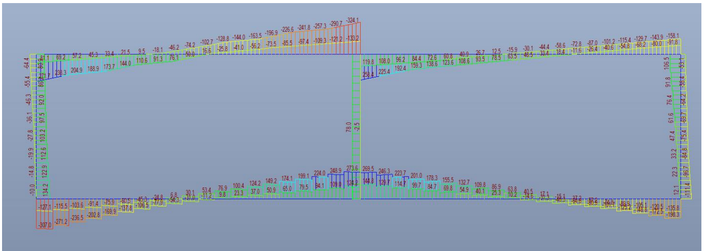
Figura 36: Involuppo SLU Taglio [kN]
