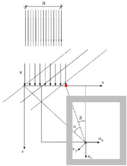
Figura 25: Formulazione di Boussinesq
