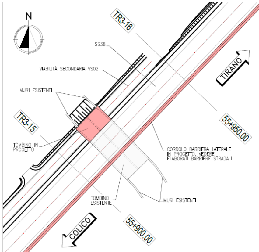
Figura 3: Vista in pianta del tombino
