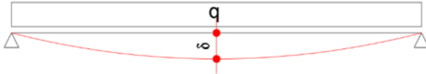
Figura 52: Massima freccia mezzeria carichi permanenti
