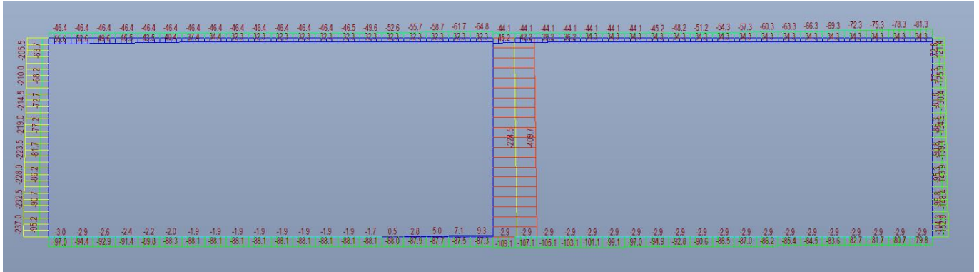
Figura 41: Involuppo SLE rara Azione assiale [kN]
